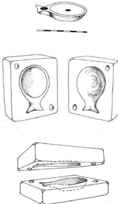
Figura 5: Desarrollo de un molde para la fabricación de lucernas (Cuomo di Caprio, 1985: 82).
