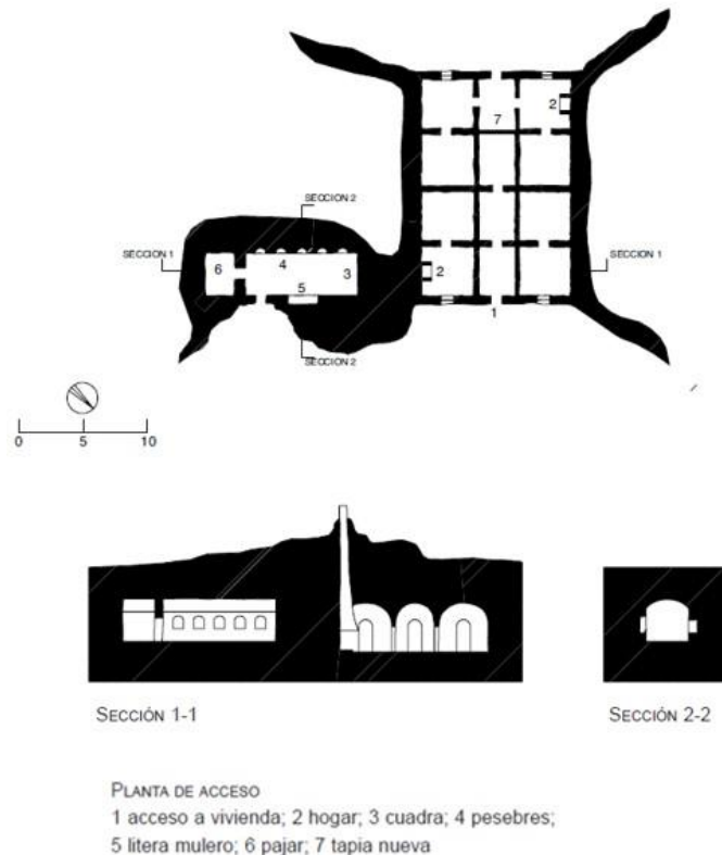
Figura 7: Plantas y secciones del Cortijo del Ceque en Fonelas Fuente: Croquis de E. Zurita Povedano (c. 1998)
