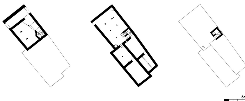
Figura 3: Plantas de la casa de Ghazouane, Alto Atlas, Marruecos Fuente: R. Costa y D. Batista (2018)
