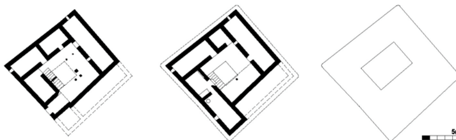
Figura 4: Plantas de la casa de Mediouna, Medio Atlas, Marruecos Fuente: R. Costa y D. Batista (2018)
