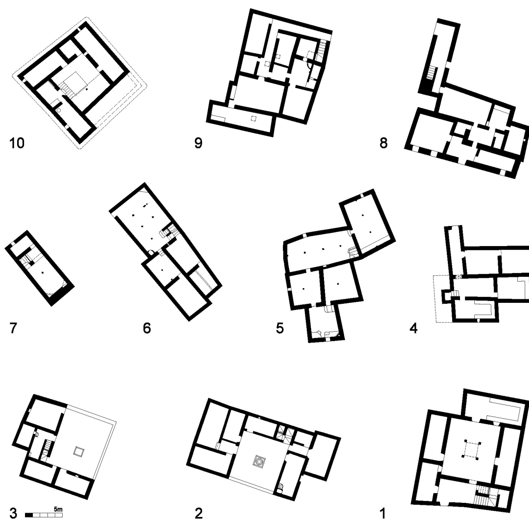
Figura 7: Plantas del piso principal de la habitación: (1-2) Ouled Yahia; (3) Ouled Sidi Ibrahim; (4) Zaouit; (5) Tameslent; (6) Ghazouane; (7) Sidi Hamza; (8/9) Zaouit; (10) Mediouna Fuente: R. Costa y D. Batista (2018)
