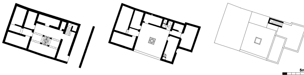
Figura 2: Plantas de la casa de Ouled Yahia, Erfoud, Marruecos Fuente: R. Costa y D. Batista (2018)
