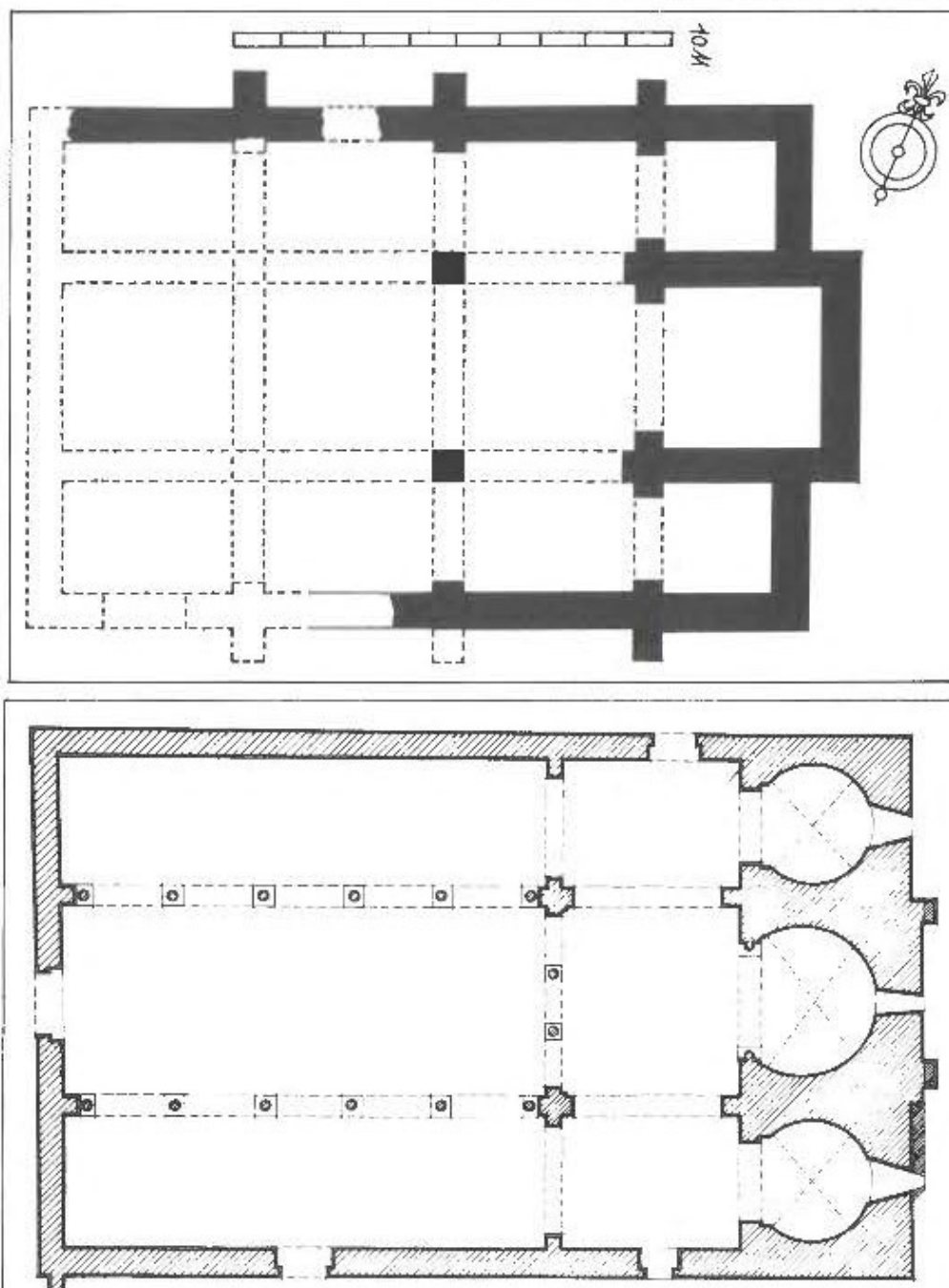
Plantas de Santa María de Bamba (arriba) y de San Miguel de la Escalada (abajo), según M. Gómez Moreno
