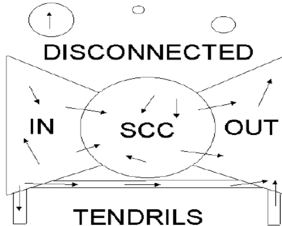
Figura 2.1. Modelo de pajarita de la Web, por Broder et al. (2000)
