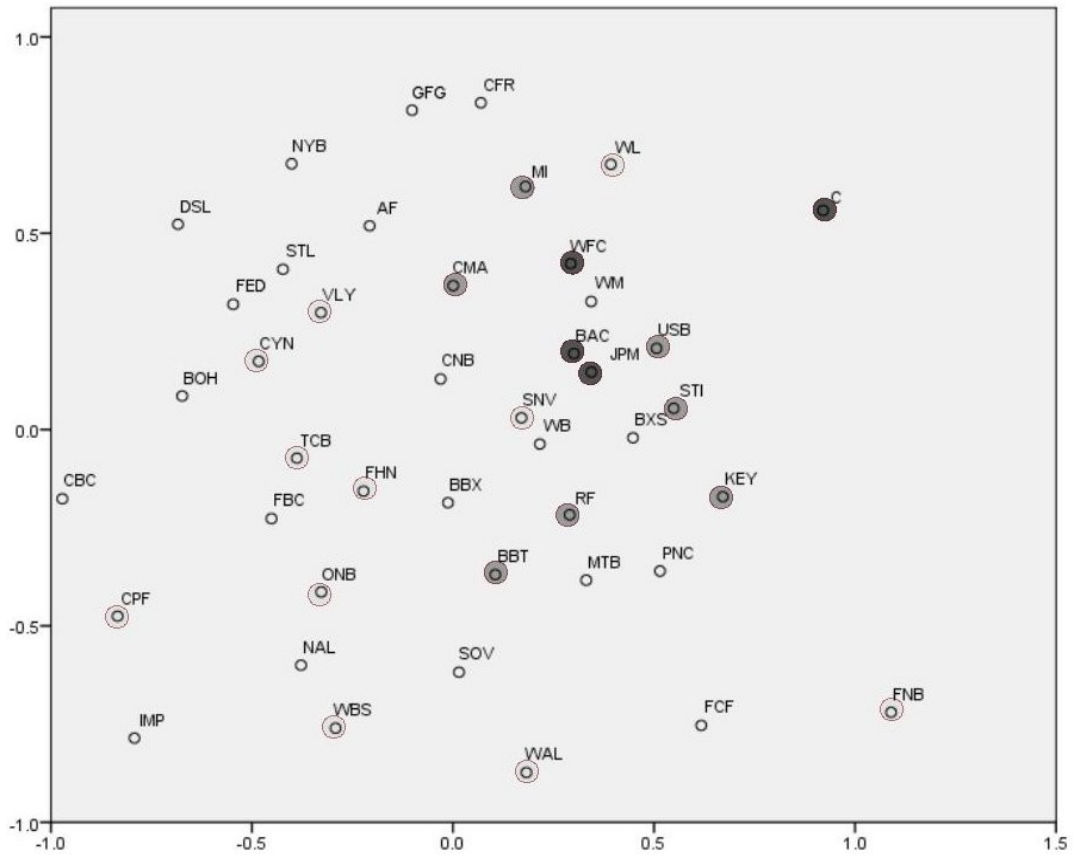
Figura 4.9. Mapa MDS sin palabras clave (enero 2009)
