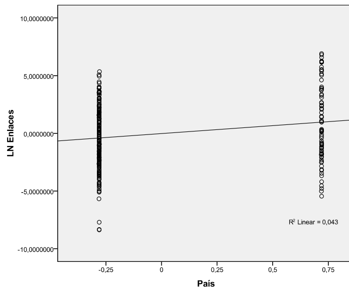
Diagramas de regresión parcial de las variables del modelo
