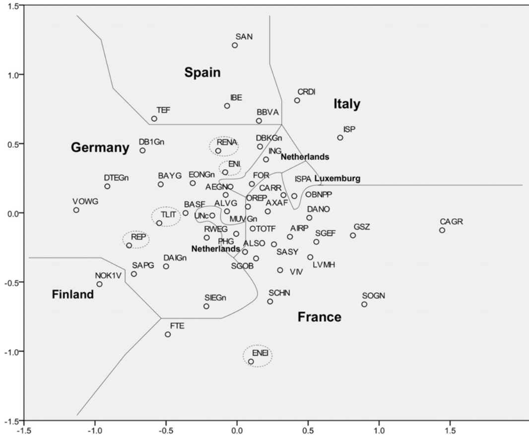
Figura 4.5. Mapa MDS del Euro Stoxx 50, con interpretación basada en países.
