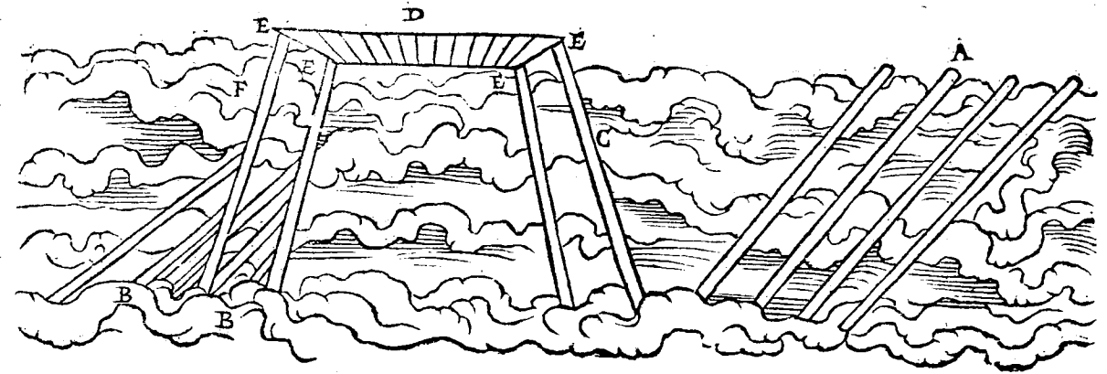
A, Sublicae superiores aduersus flumen. B B, Sublicae inferiores annexae ponti. C, Tigna bina superiora.
