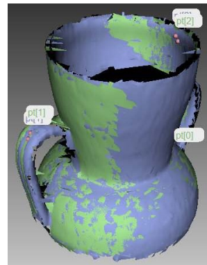
b) Registro de los scanners
