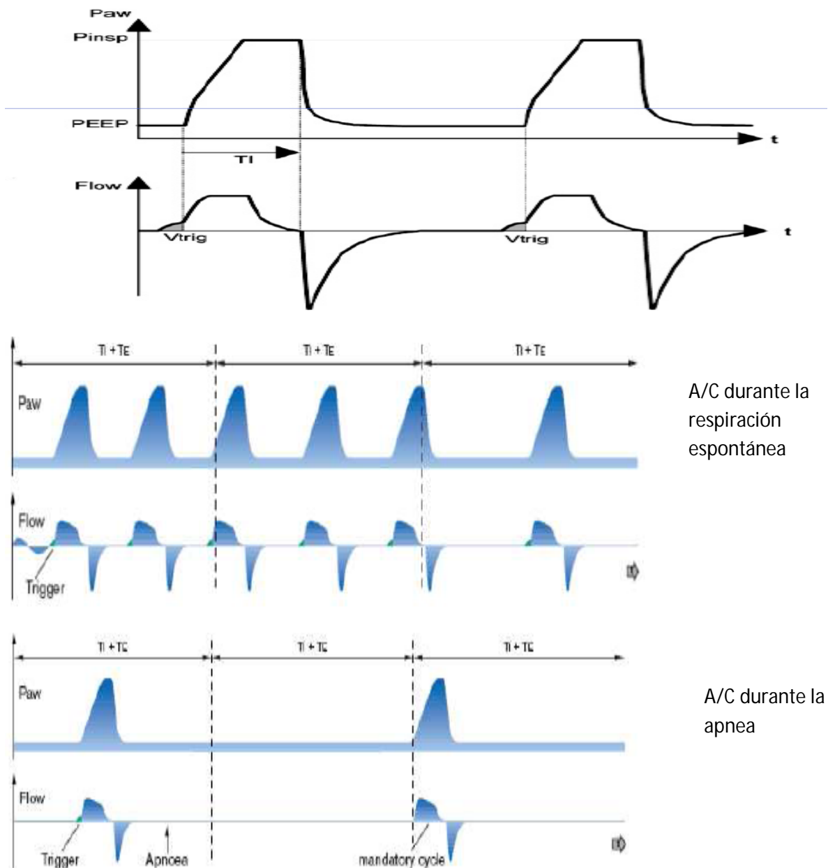
Figura 6.46. Ventilación asistida/controlada (A/C). Ondas de flujo y presión.
