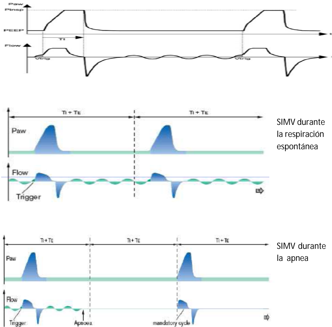
Figura 6.45. SIMV: gráficas de flujo y presión.
