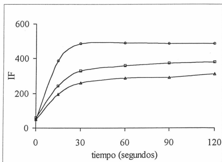
Figura III.4.2. Influencia del tiempo de agitación. fenol (□), bisfenol A (○) y BADGE (Δ).
