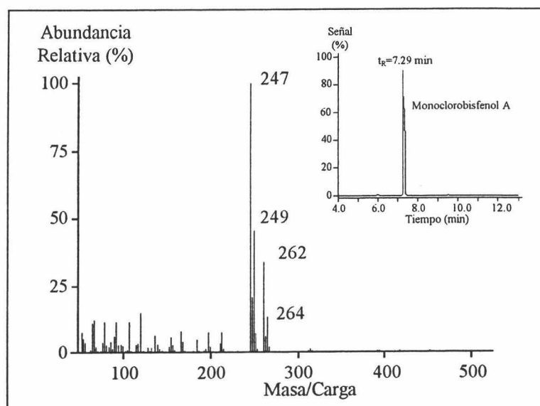
Figura IV.2.10. Cromatograma y espectro de masas del monoclorobisfenol A.
