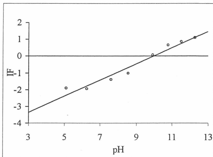
Figura III.2.6. Determinación de K_a del complejo.
