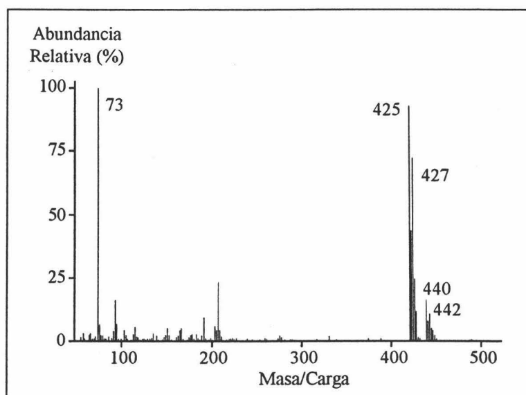
Figura IV.2.4. Espectro de masas del compuesto con t_R=8.65 min.
