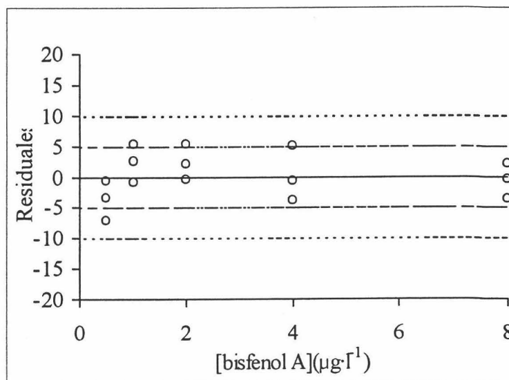
Figura III.3.13. Evaluación de la condición de homocedasticidad (500 ml)
