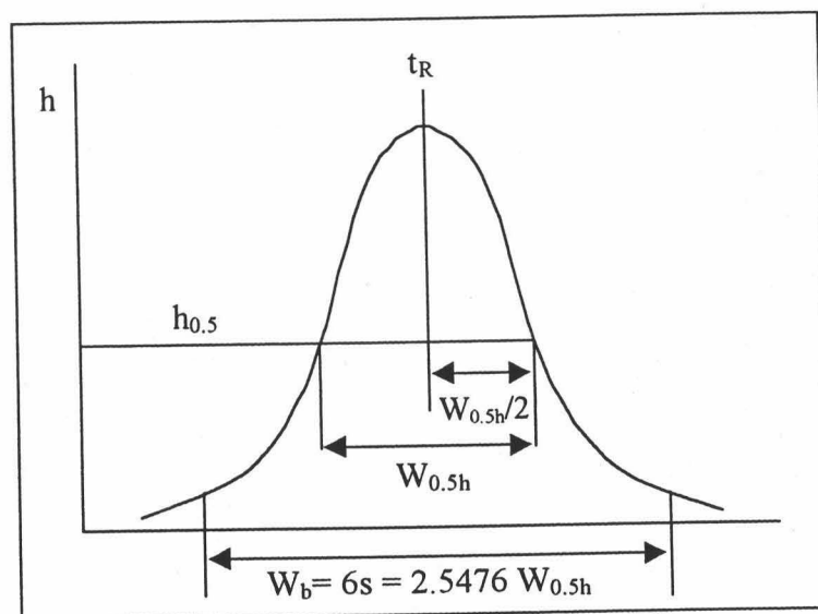
Figura II.1.2. Parámetros característicos de un pico Gaussiano.
