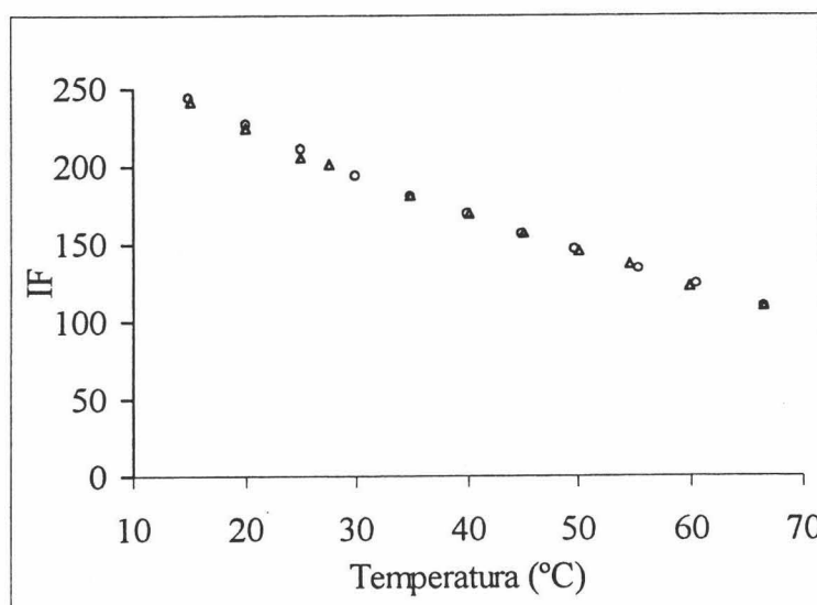
Figura III.2.8. Influencia de la temperatura: creciente (o) y decreciente (Δ).
