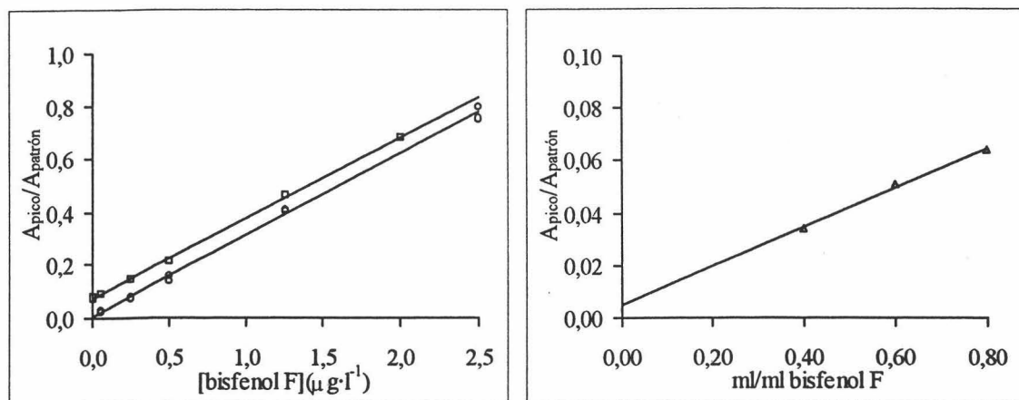
Figura IV.3.20. Calibrado con patrones (○), adición de patrón (□) y Youden (Δ) para el bisfenol F en el agua residual de la ciudad de Melilla.
