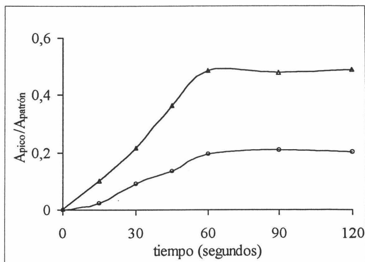
Figura IV.3.8.. Influencia del tiempo de agitación bisfenol F (○) y bisfenol A (Δ).
