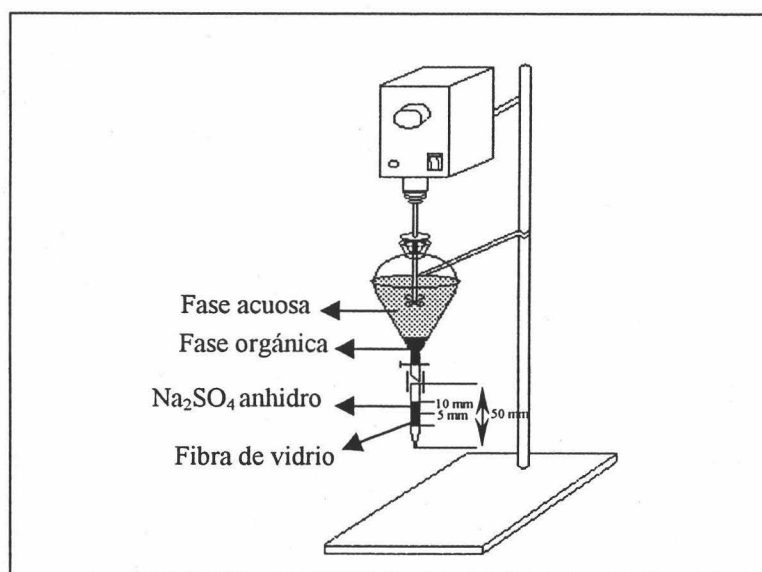
Figura III.1.6. Sistema de separación de fases para disolventes más densos que el agua.
