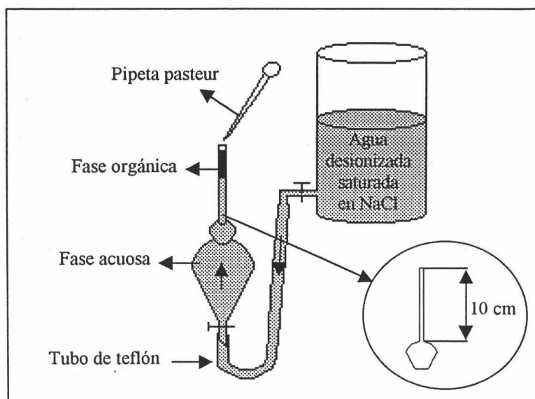
Figura III.1.7. Sistema de separación de fases para disolventes menos densos que el agua
