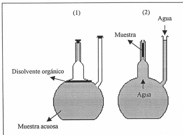
Figura III.1.2. Dispositivo de Murray.
