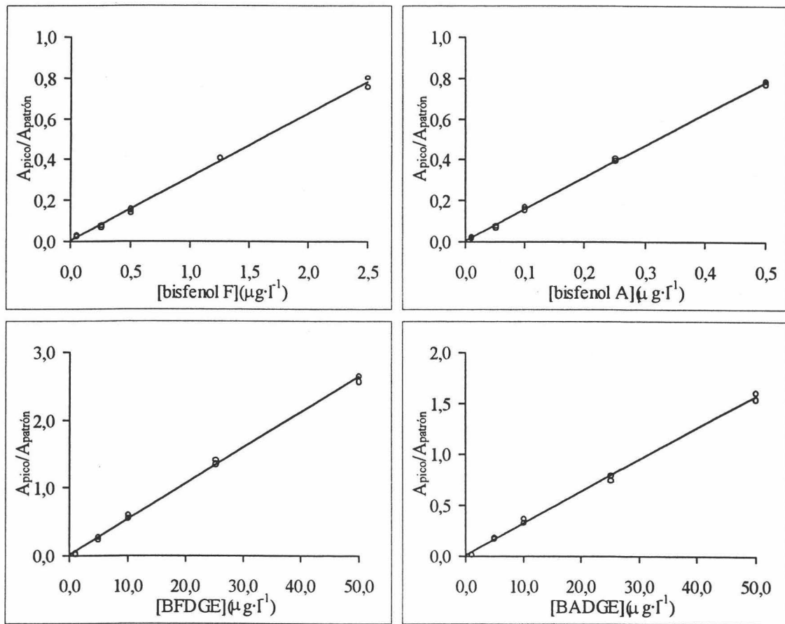
Figura IV.3.16. Calibrados con patrones.
