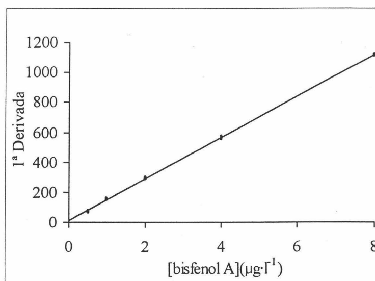
Figura III.3.10. Función de calibrado para el bisfenol A (500 ml).
