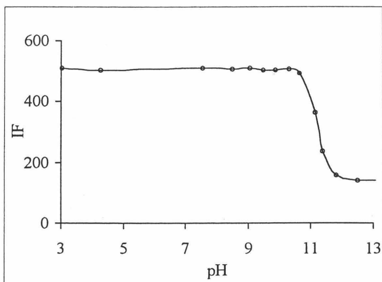
Figura III.3.6. Influencia del pH.
