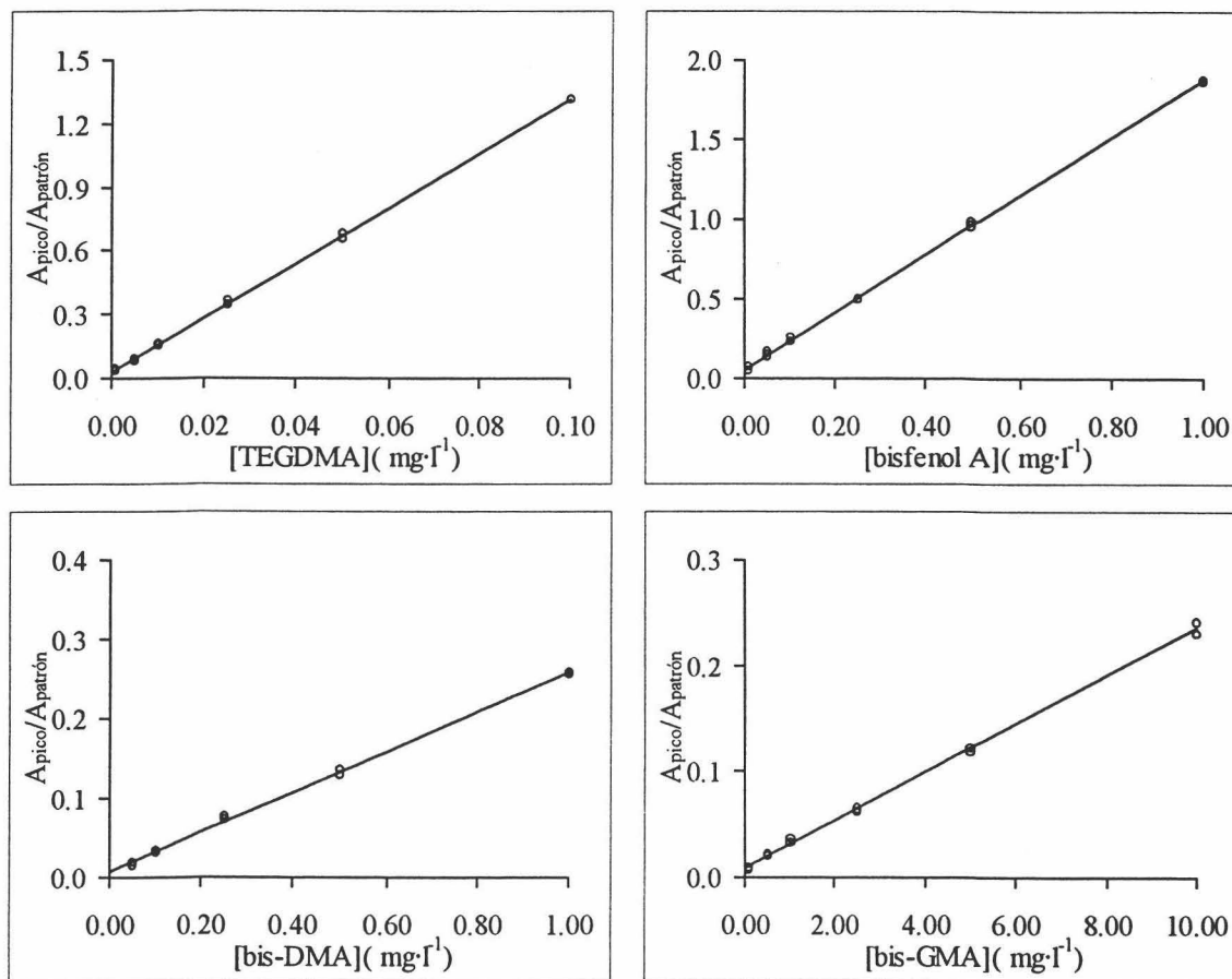
Figura IV.4.12. Calibrados con patrones.
