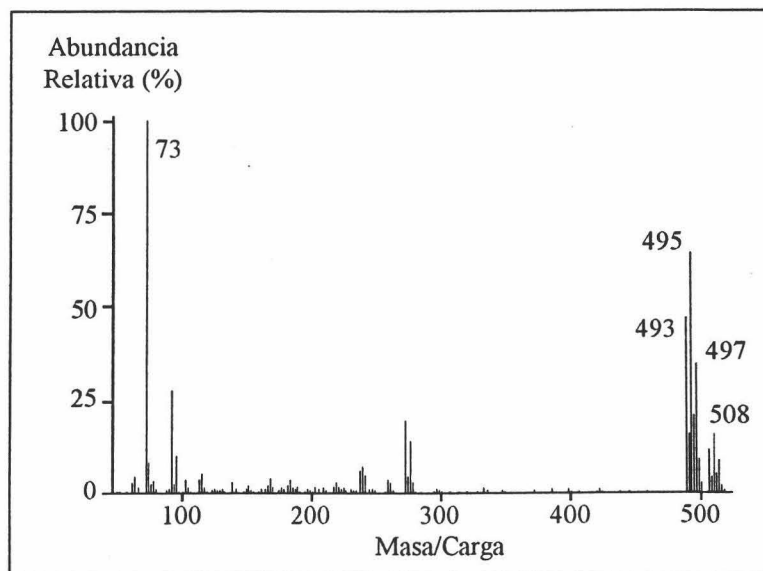
Figura IV.2.6. Espectro de masas del compuesto con t_R=10.78 min.
