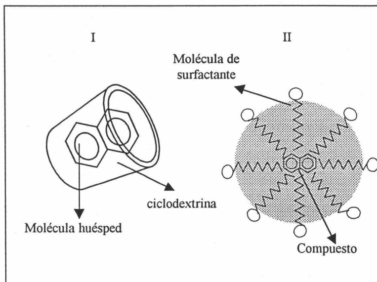
Figura III.1.1. Formación de complejos de inclusión y medios micelares.
