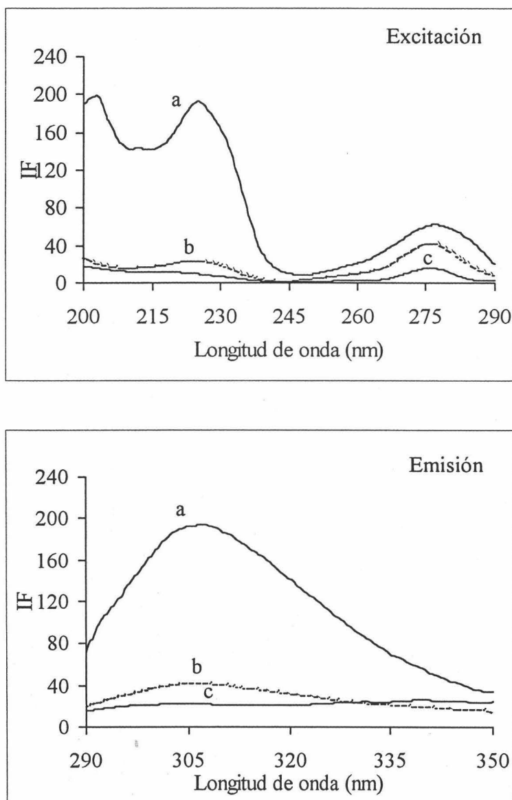
Figura III.2.1. Espectros de excitación a \lambda_{em}=306 nm y emisión a \lambda_{exc}=225 nm del bisfenol A ( 50 \mu\text{g}\cdot\text{l}^{-1} ) en presencia de \beta -ciclodextrina ( 10^{-4}\text{M} ) (a), bisfenol A en ausencia de \beta -ciclodextrina (b) y blanco (c).
