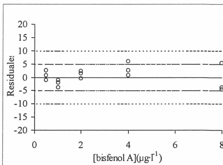
Figura III.3.12. Evaluación de la condición de homocedasticidad (250 ml)
