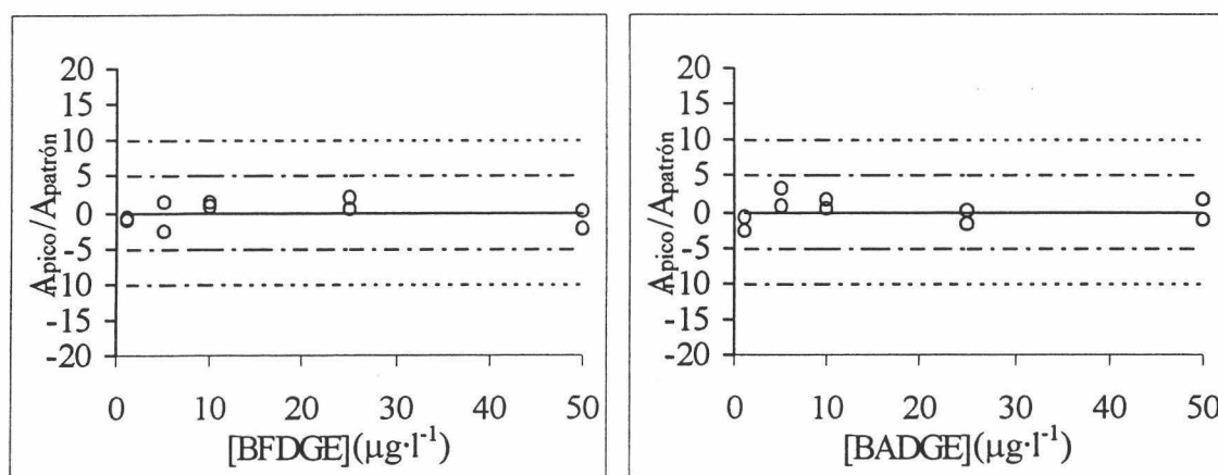
Figura IV.3.17. Evaluación de la condición de homocedasticidad.
