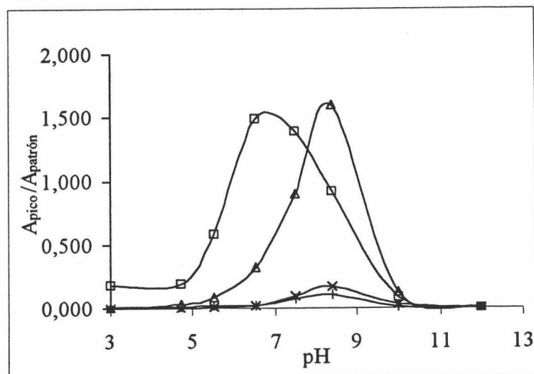
Figura IV.2.7. Evolución de la reacción con el pH bisfenol A (o), BFA-Cl ( \square ), BFA-Cl 2 ( \Delta ), BFA-Cl 3 (*), y BFA-Cl 4 (+).
