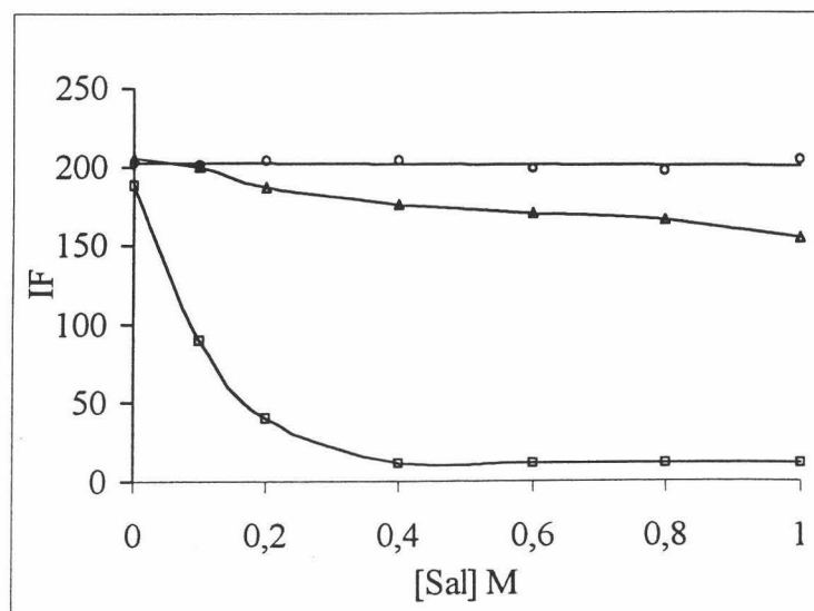
Figura III.2.7. Influencia de la fuerza iónica. NaCl (o), NaClO 4 (Δ) y CH 3 COONa (□).
