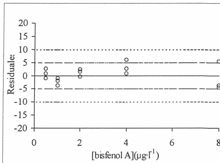
Figura III.3.11. Evaluación de la condición de homocedasticidad (100 ml)
