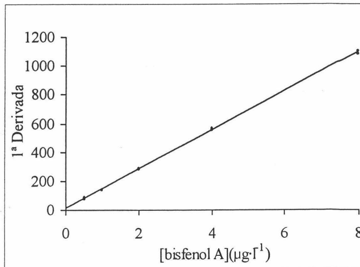
Figura III.3.9. Función de calibrado para el bisfenol A (250 ml).
