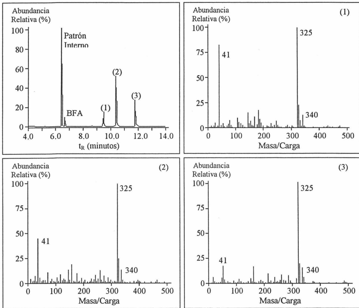
Figura IV.4.7. Cromatograma y espectros de masas del bis-GMA.
