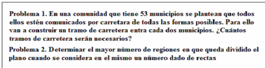
Figura 6. Problemas
