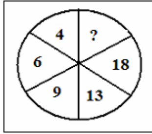
Figura 1. Círculo numérico
