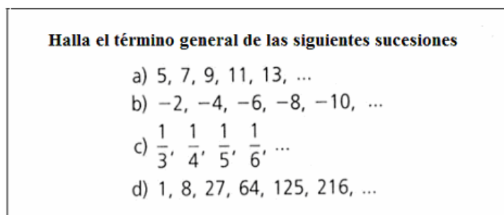
Figura 5. Sucesiones numéricas
