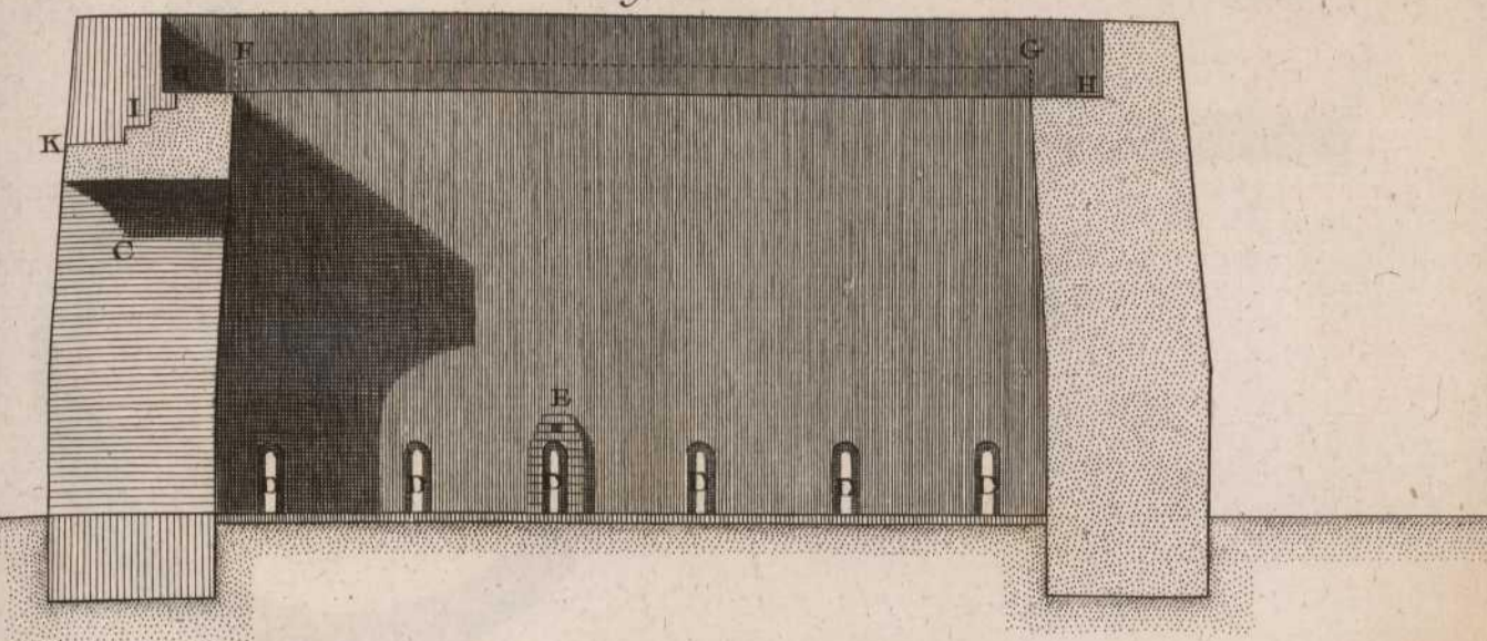
coupe sur la Ligne AB Fig. 1.
