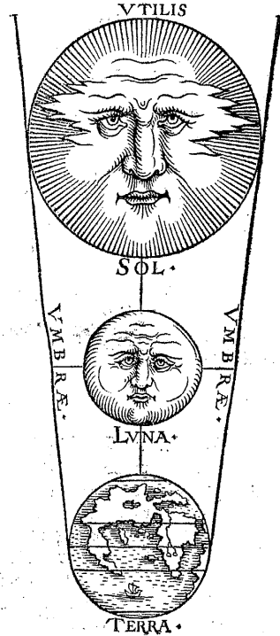
DE ECLYPSI SOLIS FIGVRA
