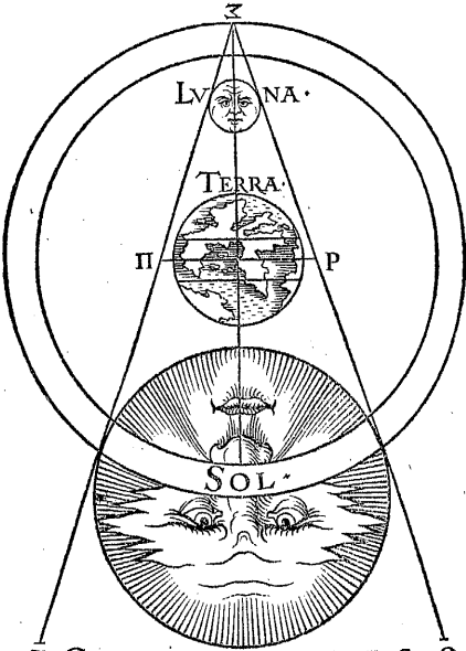
CONO IDES O
