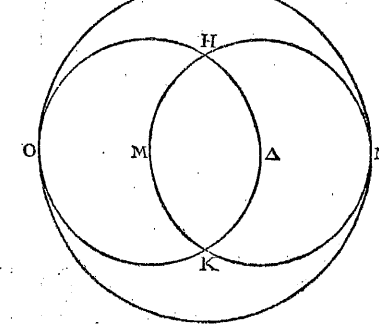
DE VNA ESSENTIA INNECTVNCVRSIBIDVO CIRCVLI.
