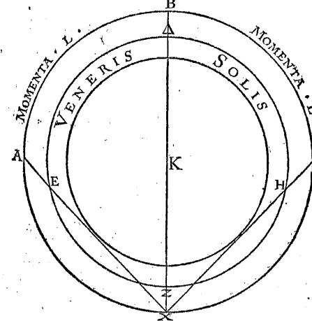
DE SOLE ET VENERE
