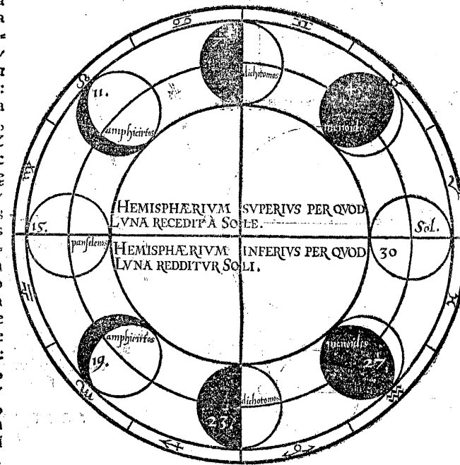
DE ECLYPSI LVNE
