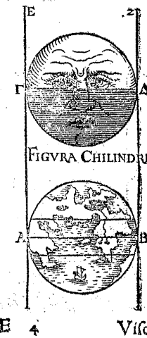
DE ECLYPSI LVNE
