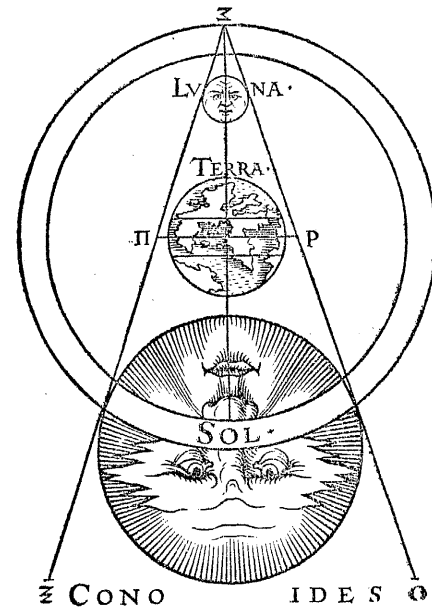
DE LVNA SOLE ET TERRA
