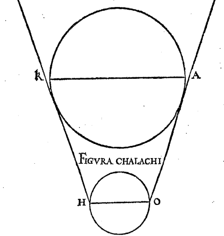
DE ECLYPSI OMIVM PLANETARVM.
