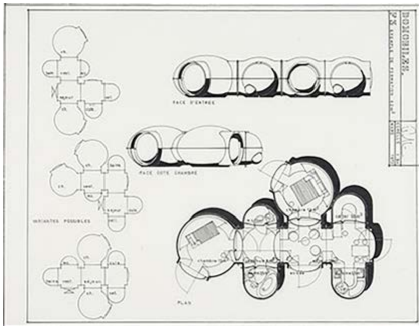
figura 3 Domobiles de Pascal Häusermann. Diseños de proyecto del prototipo: plantas, alzados, diagramas de montajes. Donación Pascal Häusermann 997 03 52 (Propiedad: François Lauginie) Colección FRAC-Centre.
