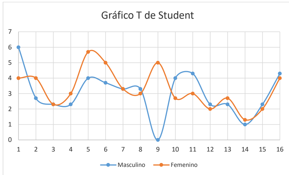
Figura 13. Gráfico T de Student
