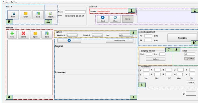
Fig. 7. FLEXOR GUI
