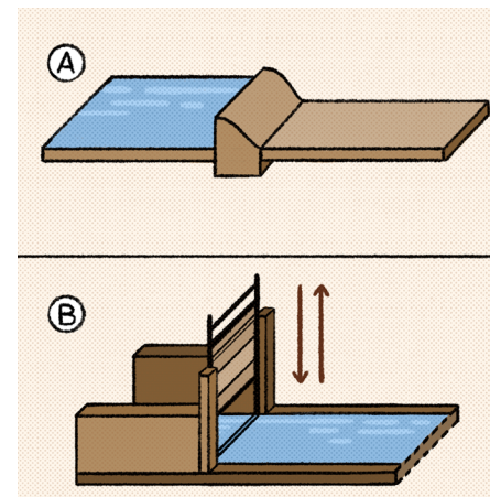
Figura 17. [A] Azud que deja seco el río. [B] Toma de agua de un canal.
