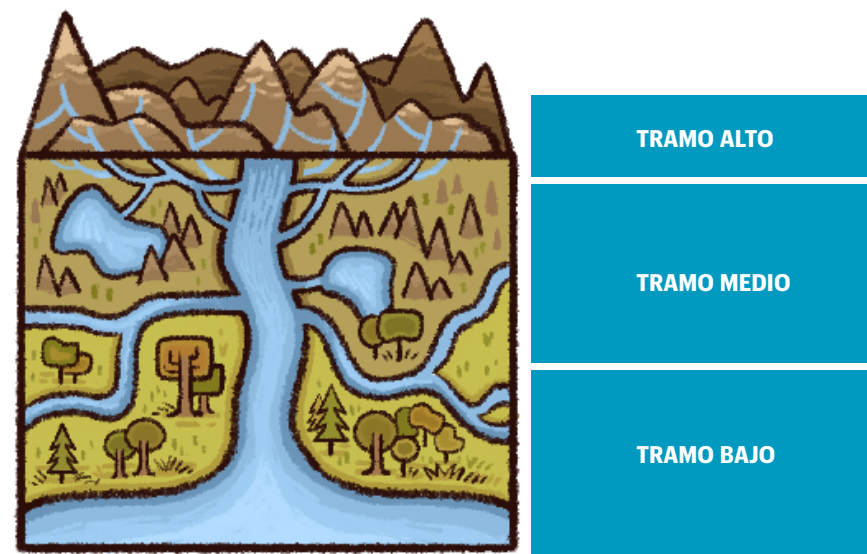
Figura 02. Tramos longitudinales de un río
