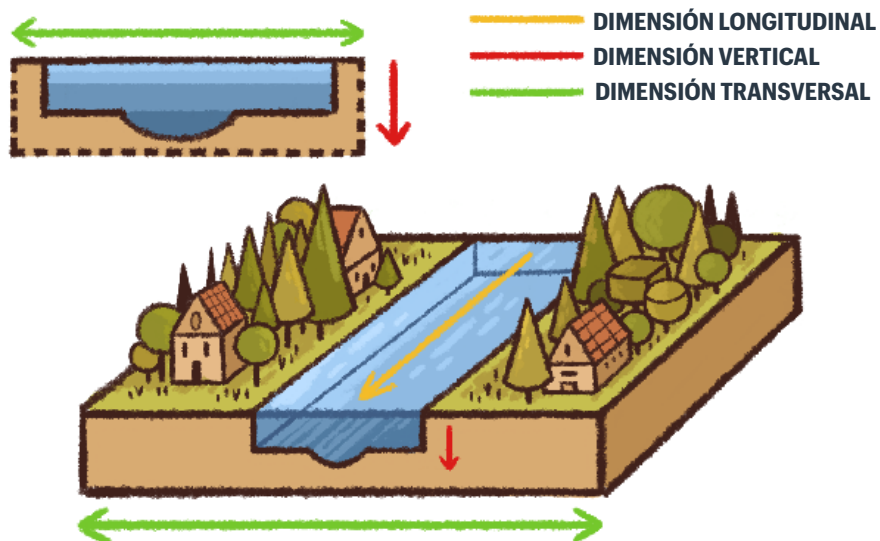
Figura 01. Dimensiones espaciales de un río
