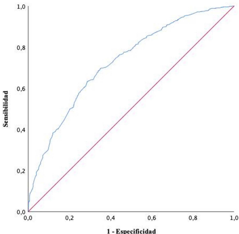
Figura 2 • Curva de rendimiento de diagnóstico (logit completo con efectos de interacción).
