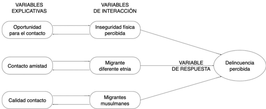
Figura 1 • Diagrama de variables para el análisis.
