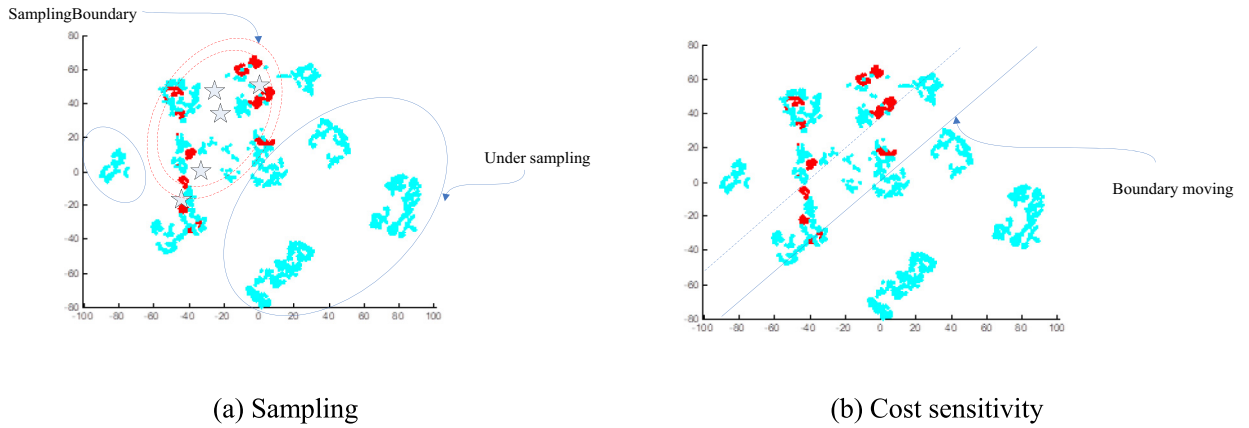
Fig. 2. Segment0.
