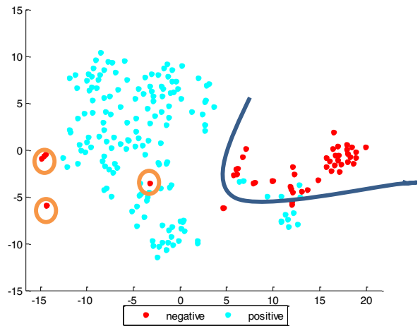
(d) Glass
