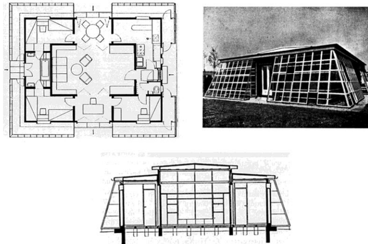
Figura 7: Martin Wagner y Leberecht Migge, Planta, sección y maquetas del proyecto wachsende Haus Fuente: Martin Wagner. Das wachsende Haus: ein Beitrag zur Lösung der städtischen Wohnungsfrage= The Growing House (Leipzig: Spector Books, 2015), 149
