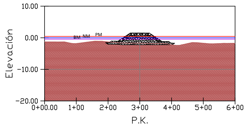
SECCIÓN 7
