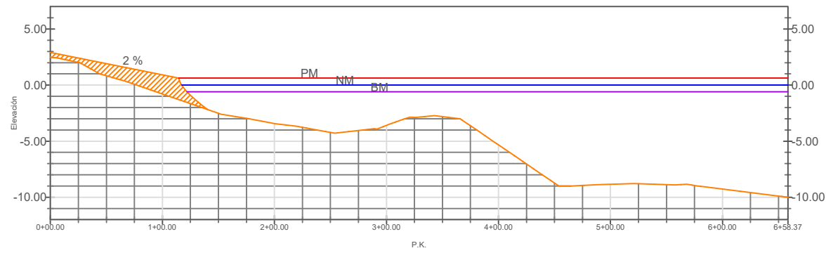
PERFIL - (15)
