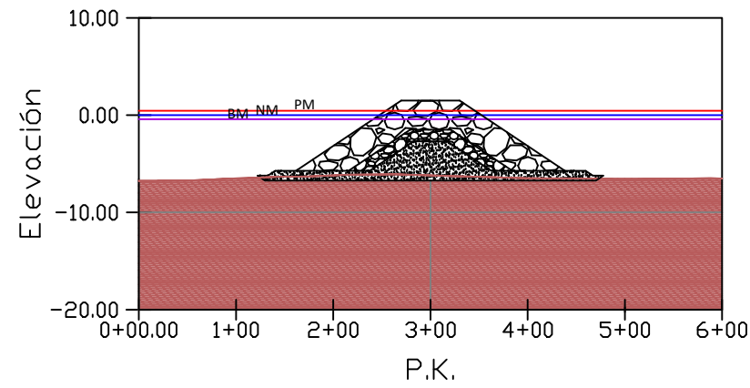
SECCIÓN 5
