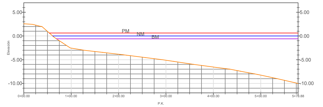
PERFIL - (19)
