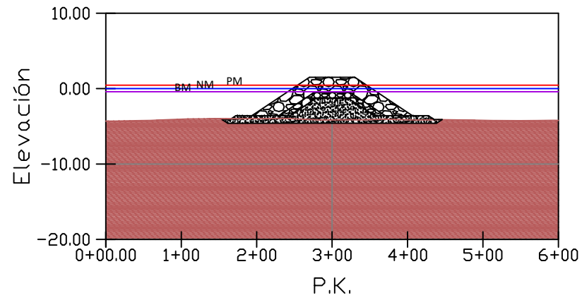
SECCIÓN 7
