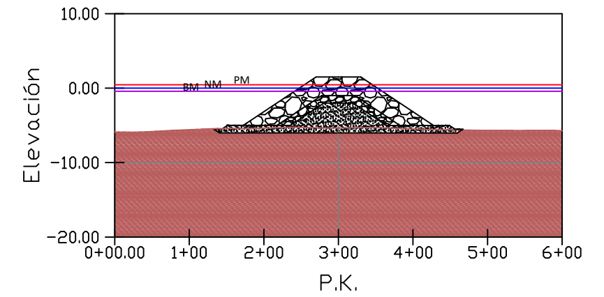
SECCIÓN 6
