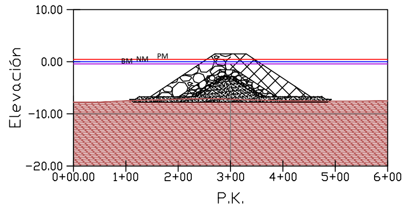
SECCIÓN 4
