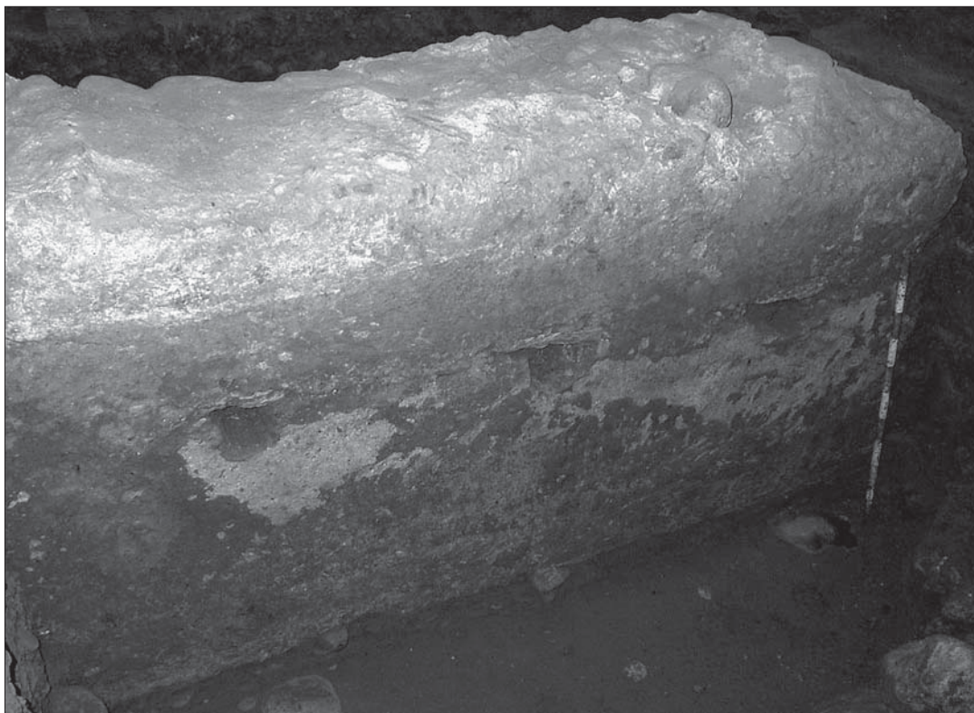
Lám. 3. Muro de tapial de calicanto del recinto residencial zirí.
