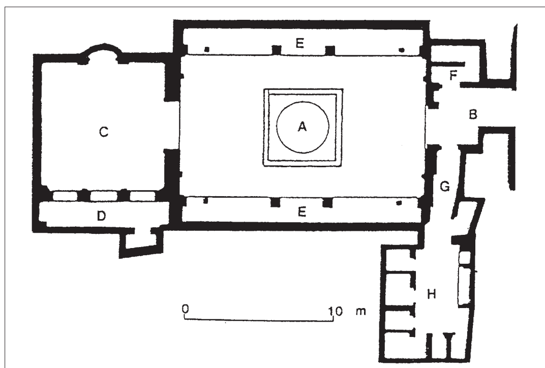
Lám. 8. Planta de la madrasa al-'Aṭṭārīn de Fes (GOLVIN, 1995: 230).
