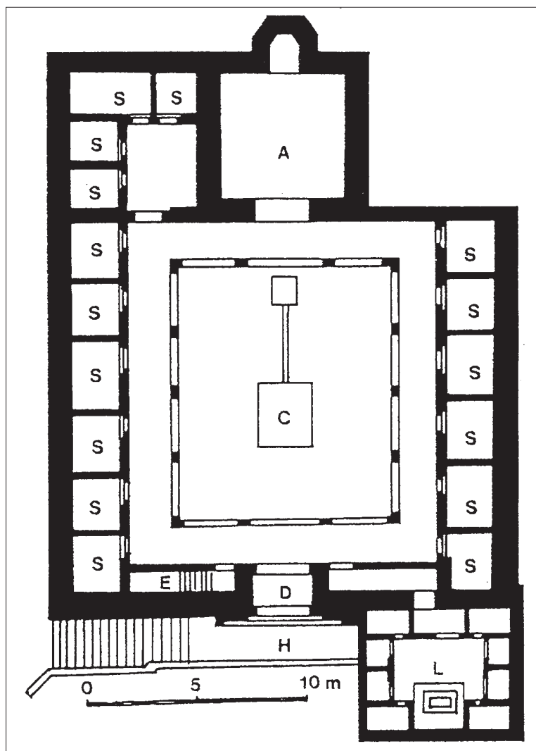
Lám. 7. Planta madrasa al-'Ubbād de Tremecén (GOLVIN, 1995:203).
