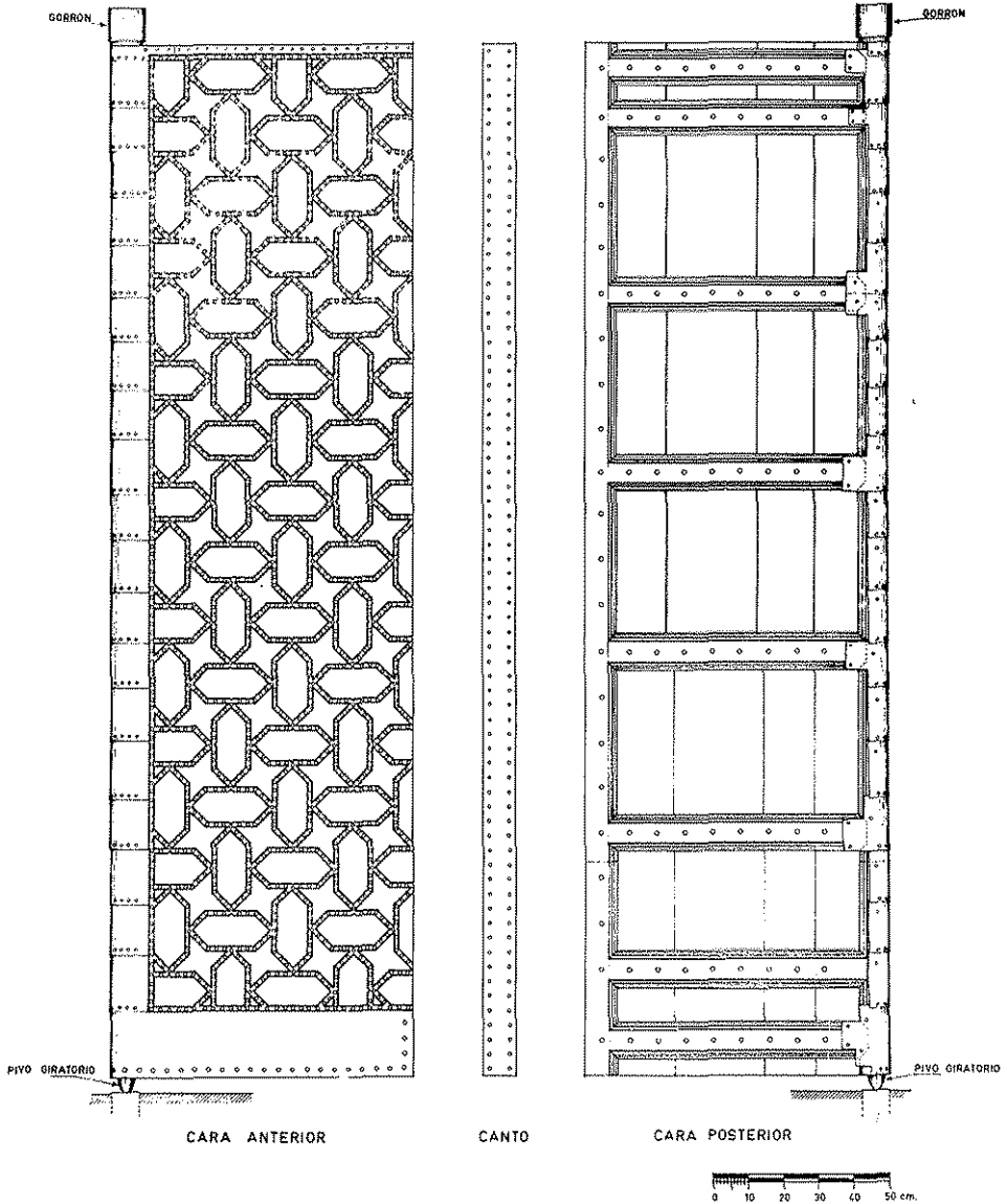
Figura 3.—Hoja original de la fachada de Comares restaurada (dibujo: M. López Reche)
