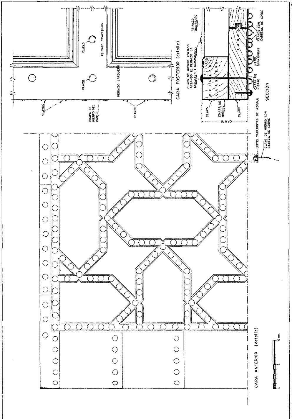
Figura 4.—Detalle de la traza y peinacería de la puerta (dibujo: M. López Reche)
