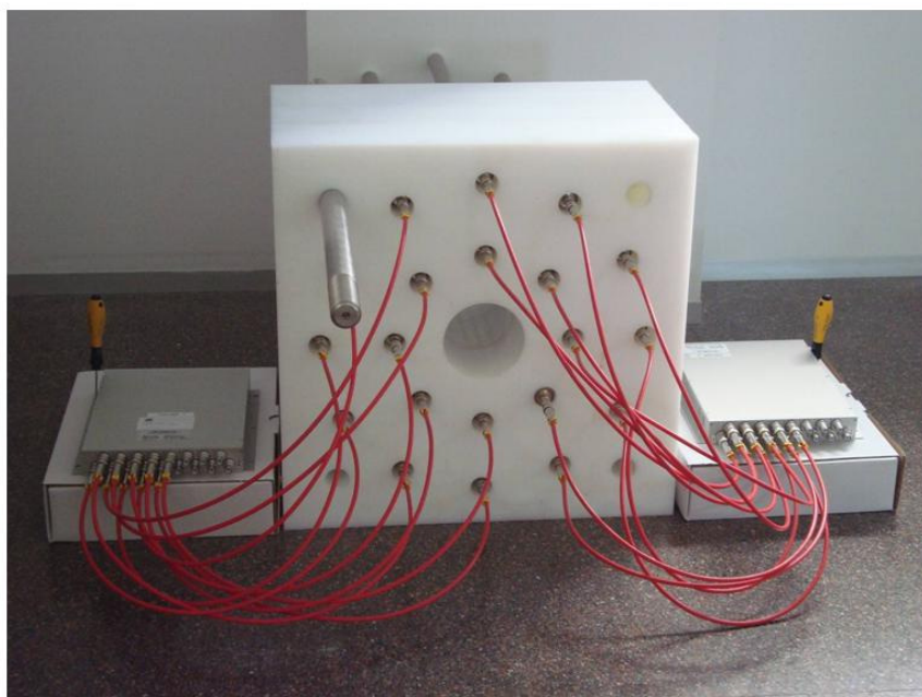
Figure 77: 4\pi neutron detector prototype assembled at the Universitat Politècnica de Catalunya lab.
