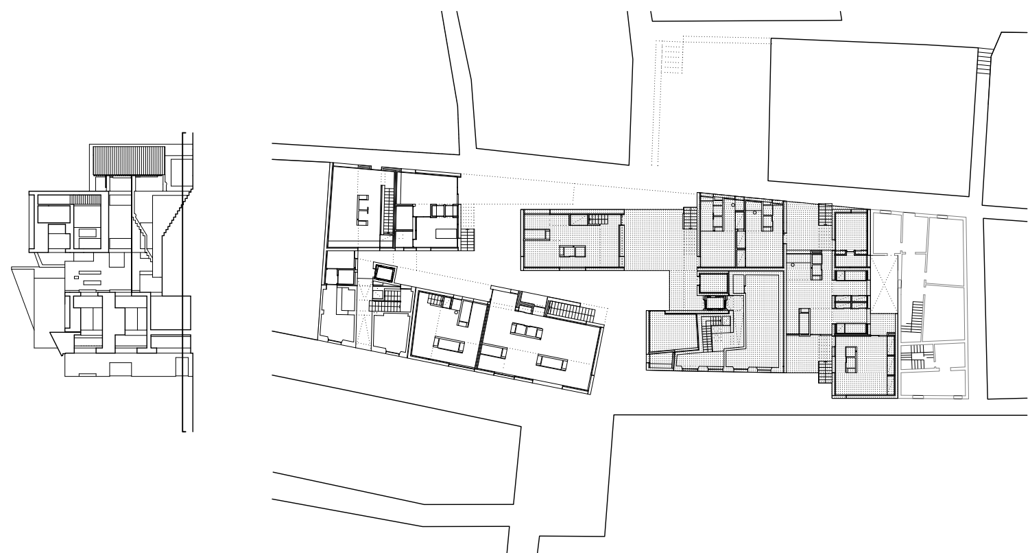
PLANTA NIVEL +0.00
