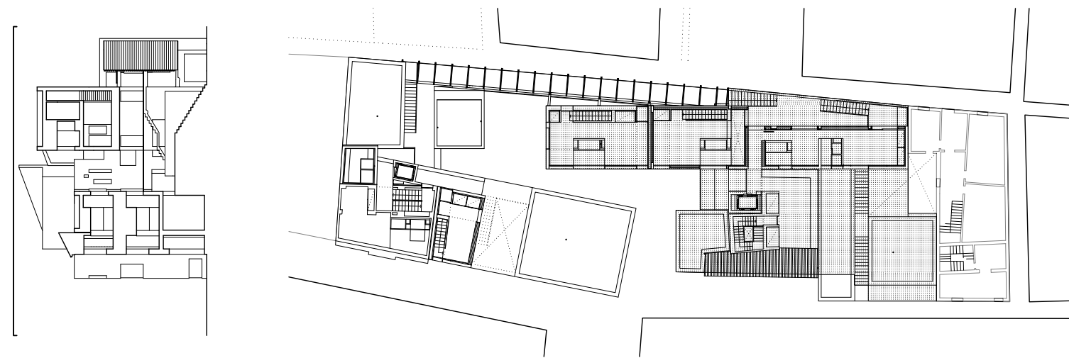
PLANTA NIVEL + 11.84
