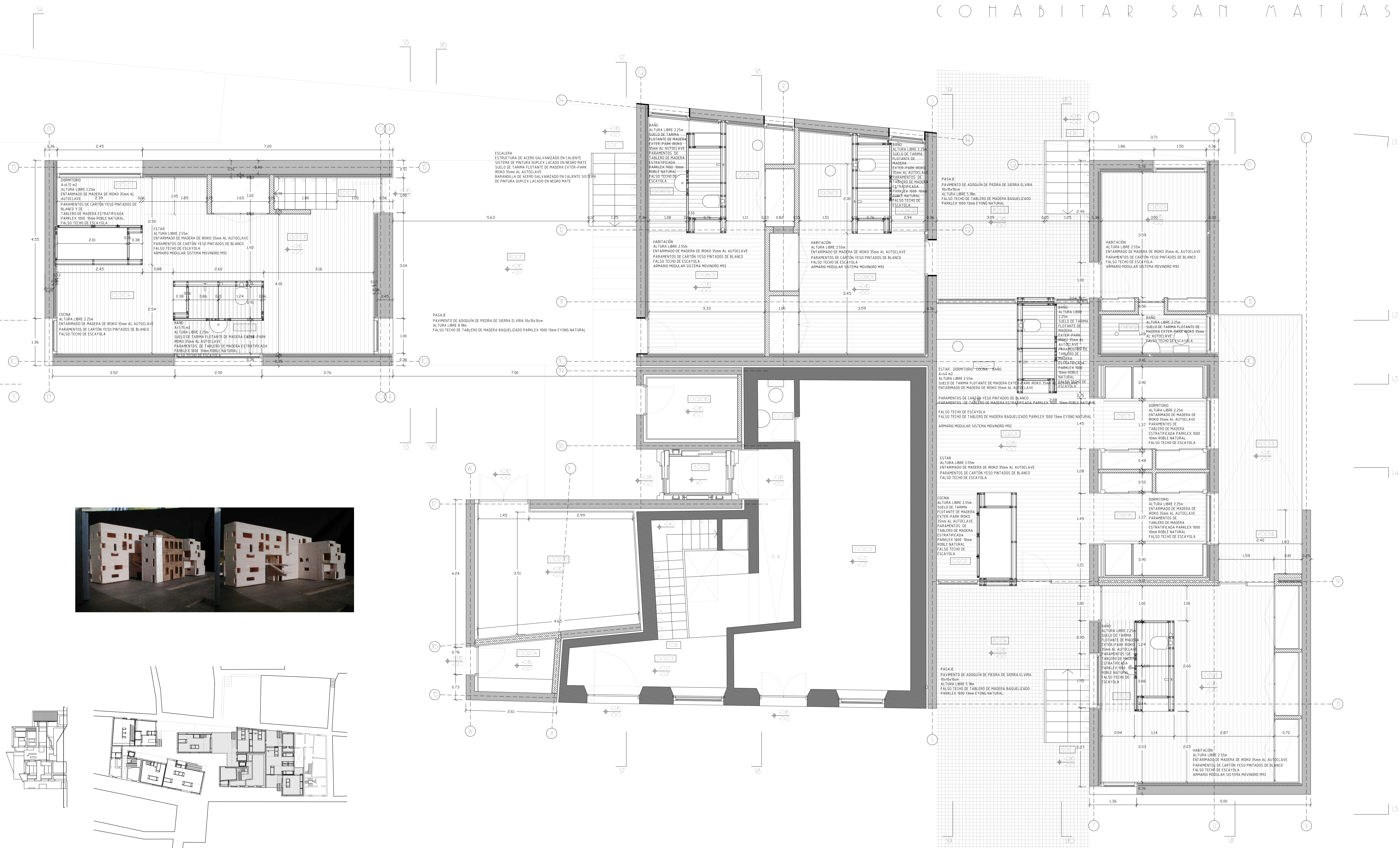
PLANTA NIVEL +0.00
