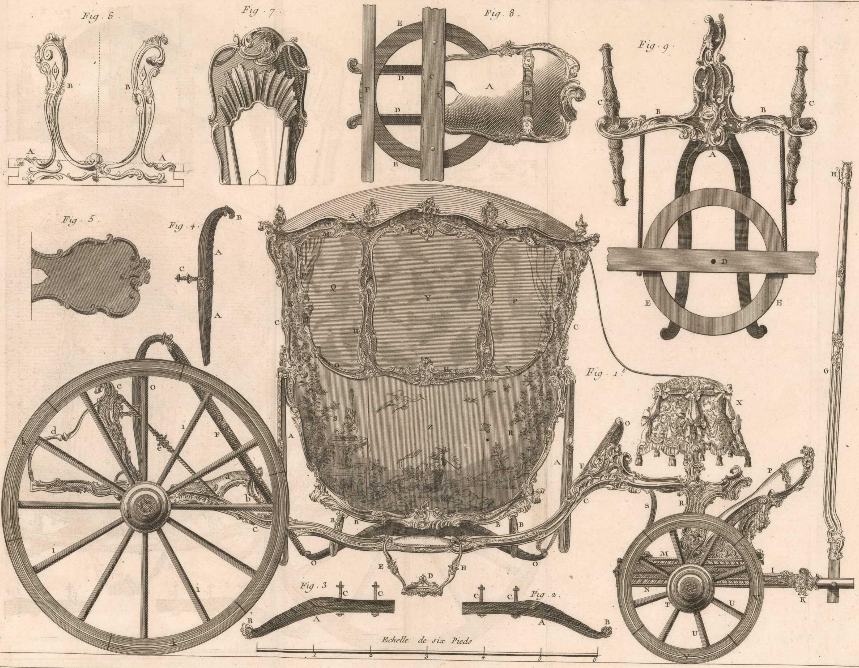
Sellier-Carrossier, Berline ou vis-à-vis à panneaux arrasés.
