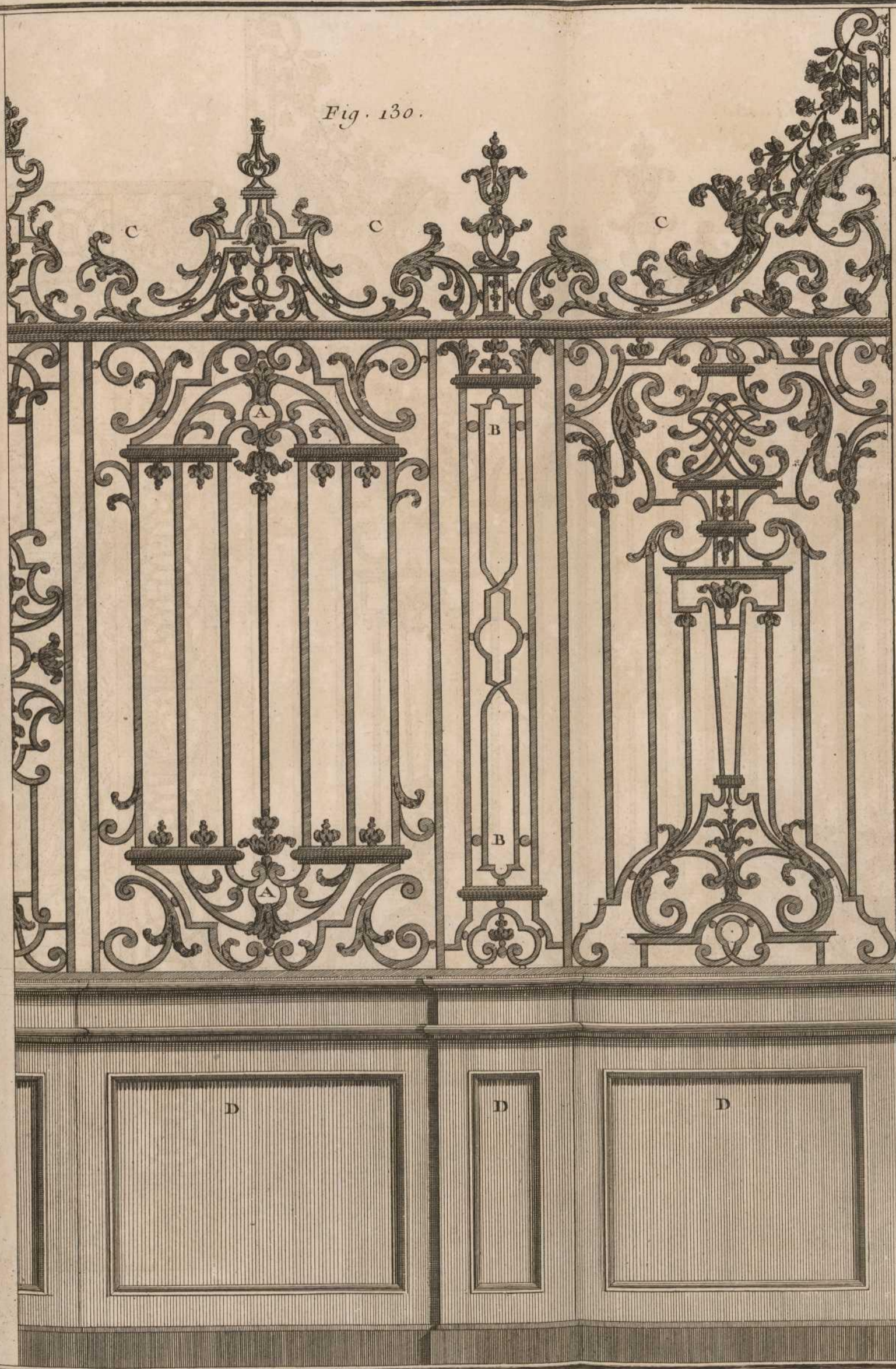
Serrurerie, Grands Ouvrages, Grilles Battante et Dormante
