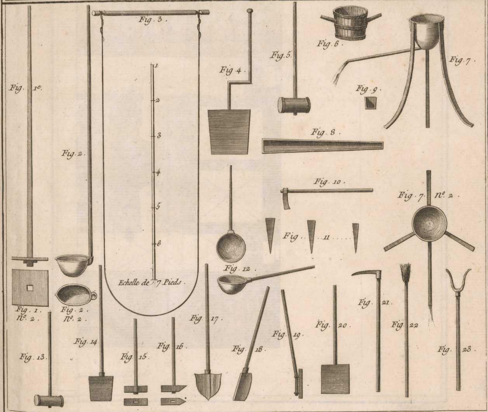
Savonnerie, Differentes Operations pour la preparation du Savon et Ustenciles.
