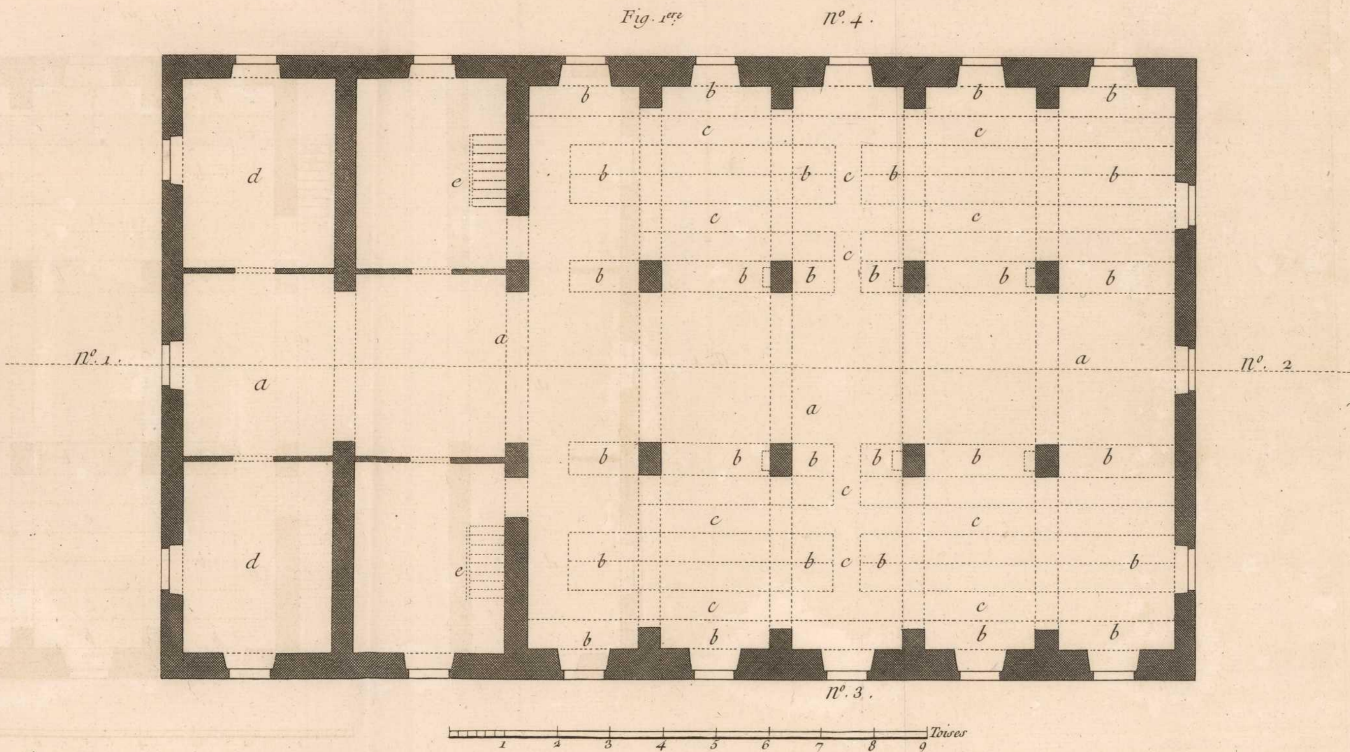
Savonnerie, Plan du premier Etage d'une Manufacture de Savon, et Operations pour partager egallement et couper le Savon.
