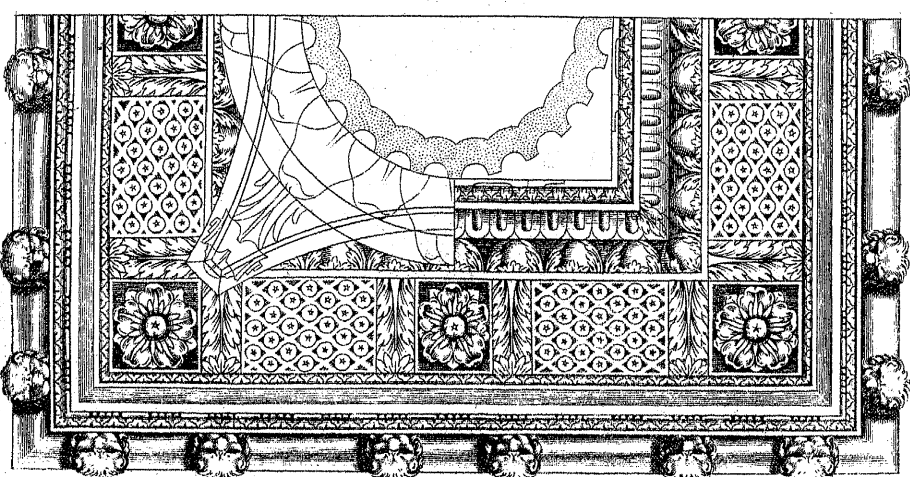
SACRAE ARCHITECTVRAE PARTES EARVMQVE MENSVRAE ET ORNAMENTA
