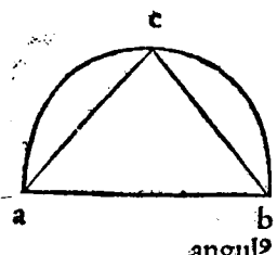
angulus in semicirculo descriptus, rectus est. quod existerectus est.
