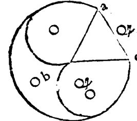
Bocardo per impossibile.
