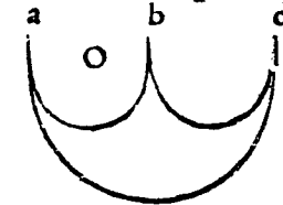
Propositio, elemētū est: assumptionem monstrat Euclides 30 tertij.
