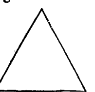
Aequilaterus Aequilater Isopleurus
