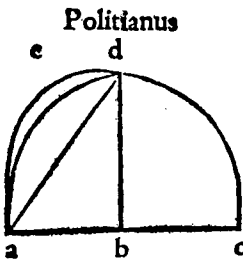
Figura a e d circumferentiarum partibus a d, & a e d: meniscus, lunulæque dicitur.
