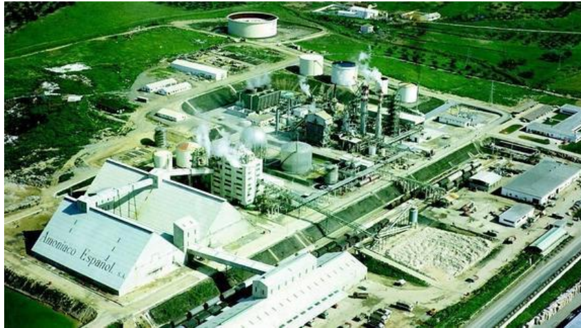
Figura 2: Planta de Amoniaco Español, S. A. (Málaga).
