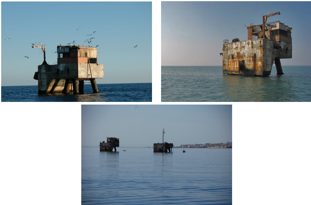
Figura 1: Pantalán de Cros-Amonesa (costa de Málaga).
