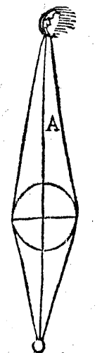
Corona ratio.
