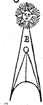
Arcus ratio.
