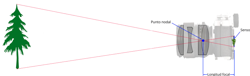
Figura 2.8: Relación entre el punto nodal y la distancia focal en un sistema óptico [55]. La imagen muestra cómo la luz que pasa por el punto nodal de la lente converge en el sensor de la cámara.
