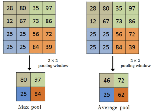
Figura 2.6: Tipos de pooling comúnmente utilizados en CNN [48]. En el max pooling , se selecciona el valor máximo de una región local de la matriz de características de entrada, mientras que en el average pooling , se calcula el promedio de los valores en una región local.
