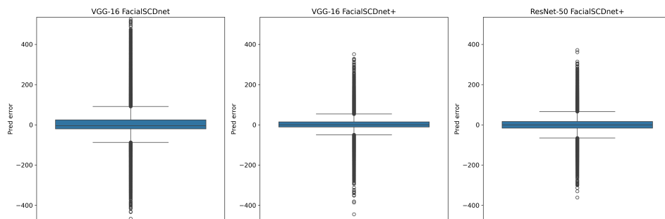
Figura 5.2: Gráfica que muestra la comparación de las predicciones de error para cada uno de los 3 modelos utilizados.
