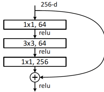
Figura 4.16: Bloque bottleneck construido para las ResNet-50/101/152 [78]. Este bloque consiste en tres capas de convolución: una convolución 1x1 que reduce la dimensionalidad a 64 canales, seguida de una convolución 3x3, que aprende las características espaciales, y otra convolución 1x1 que restaura la dimensionalidad original de 256 canales. Todas las capas de convolución usan activaciones ReLU. La conexión de salto agrega la entrada del bloque directamente a la salida, antes de pasar por una activación ReLU final.
