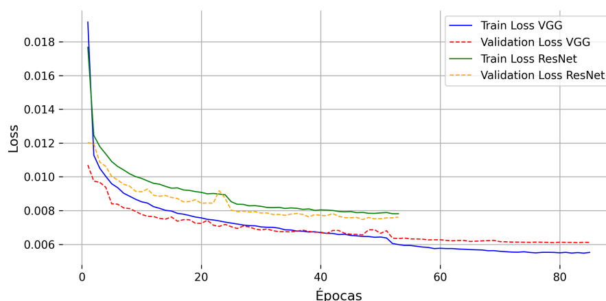
Figura 5.1: Gráfica de la función de pérdida durante el entrenamiento de las redes VGG-16 y ResNet-50. Para la red VGG se representa en azul la pérdida en el conjunto de entrenamiento mientras que en rojo se representa la pérdida en el conjunto de validación. Para la red ResNet se representa en verde la pérdida en el conjunto de entrenamiento mientras que en naranja se representa la pérdida en el conjunto de validación.
