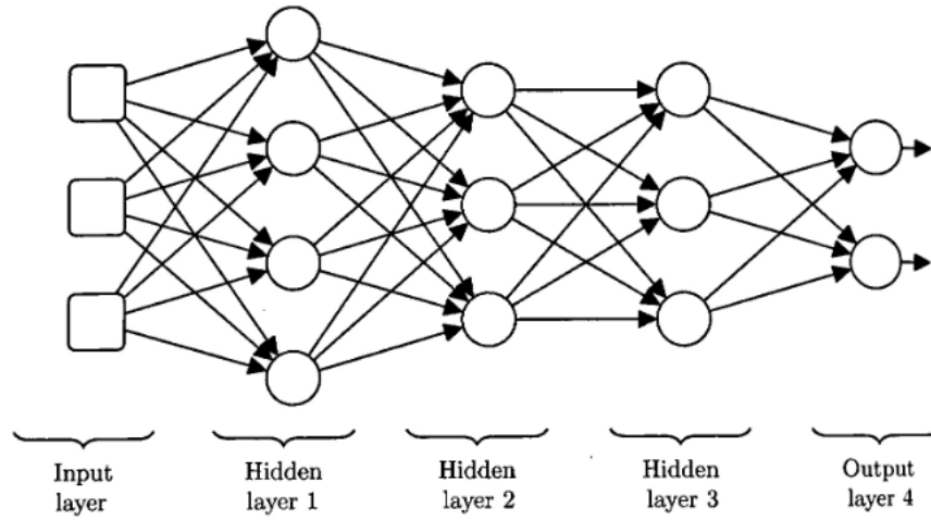
Figura 2.1: Esquema general de una red neuronal [37], que consta de una capa de unidades de entrada, una capa de unidades de salida y tres capas de unidades ocultas. Cada círculo representa una unidad de procesamiento simple, la cual incluye el producto escalar de pesos por entradas y una función de activación (generalmente no lineal), tal como se muestra en la Figura 2.2.
