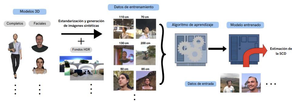
Figura 1.3: Diagrama del proceso de estimación automática de la SCD en este proyecto. El punto de partida es una serie de modelos 3D, tanto completos como faciales, a los cuales se les aplicará un proceso de estandarización y normalización. Posteriormente, se añadirán fondos HDR para generar imágenes fotorrealistas a diferentes distancias, las cuales se utilizarán para entrenar el modelo de aprendizaje con el objetivo de estimar la SCD ante nuevos datos de entrada.
