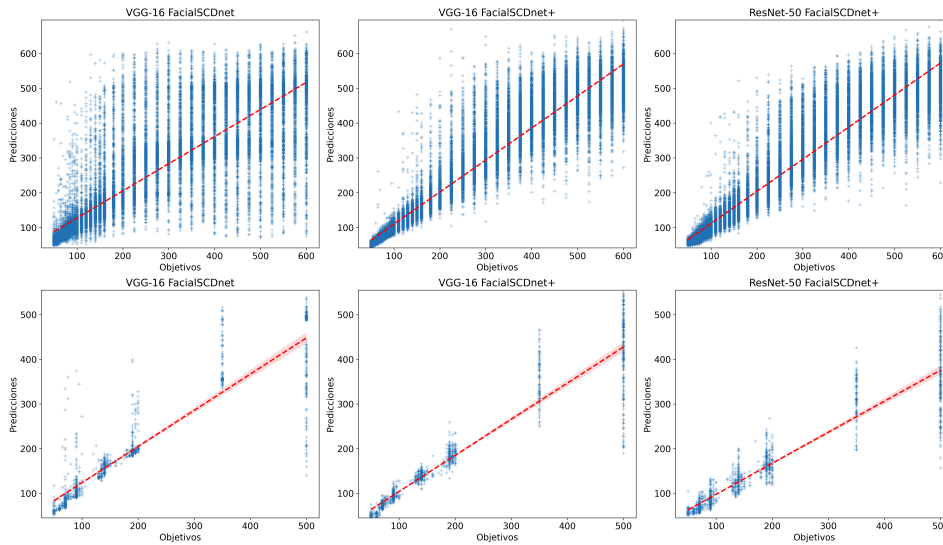
Figura 5.6: Gráfica comparativa de predicciones vs objetivos para los tres modelos utilizados. La primera fila presenta los resultados en el conjunto de test sintético, mientras que la segunda fila muestra los resultados en el conjunto de test real.
