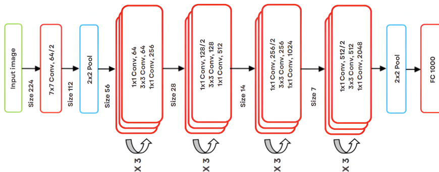
Figura 4.17: Arquitectura de la red ResNet-50 [78].
