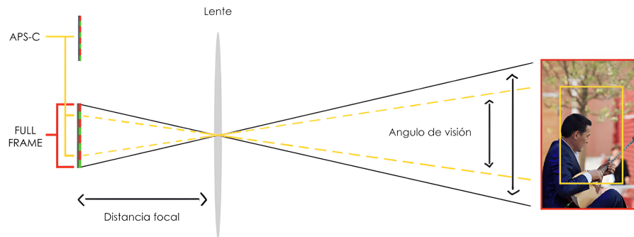
Figura 2.11: Diagrama que muestra el concepto de distancia focal equivalente en función del tamaño del sensor [58]. Se observa cómo un lente proyecta la luz en sensores de diferentes tamaños (APS-C y Full Frame), lo que modifica el ángulo de visión y, en consecuencia, la cantidad de escena capturada en la imagen resultante.
