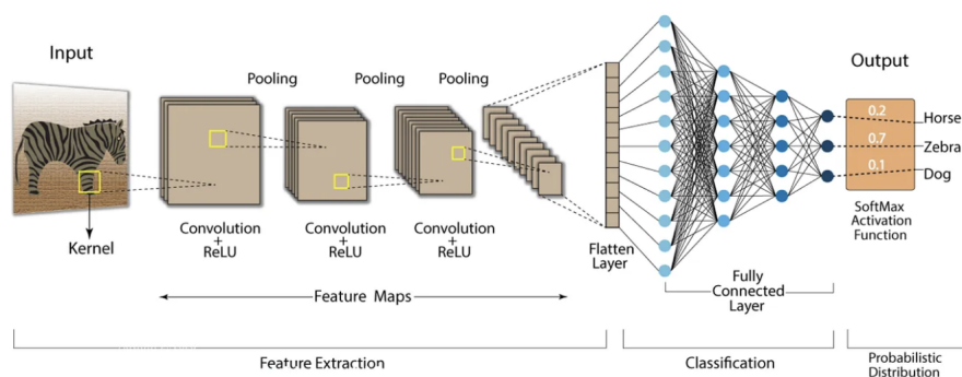
Figura 2.3: Arquitectura típica de red neuronal convolucional [45], utilizada principalmente para la tarea de clasificación de imágenes. La entrada es una imagen de un objeto. La red consta de varias capas de convolución seguidas por funciones de activación y capas de pooling que reducen la dimensionalidad de los mapas de características. Finalmente, las características extraídas se aplanan y se pasan a través de capas totalmente conectadas que terminan en una capa de clasificación softmax , proporcionando una distribución de probabilidad sobre las posibles clases de salida.
