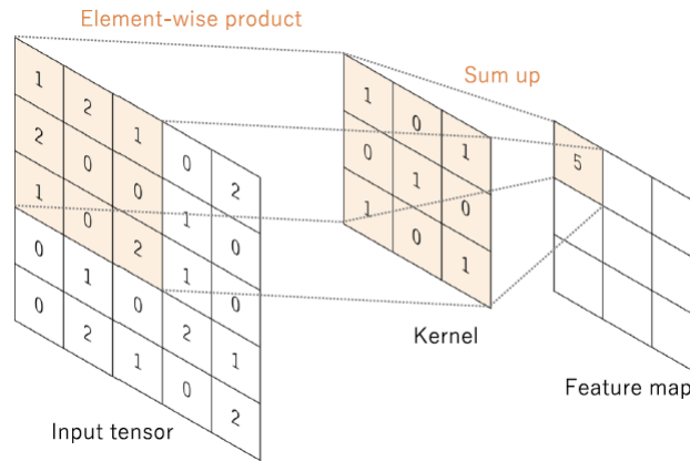
Figura 2.4: Ejemplo de operación de convolución en CNN [47]. Se muestra cómo un kernel se aplica sobre un tensor de entrada (una matriz de píxeles de la imagen), realizando un producto elemento a elemento. Los productos resultantes se suman para obtener un único valor en el mapa de características. Este proceso se repite para cada posición del kernel sobre la imagen de entrada, generando así un nuevo mapa de características.
