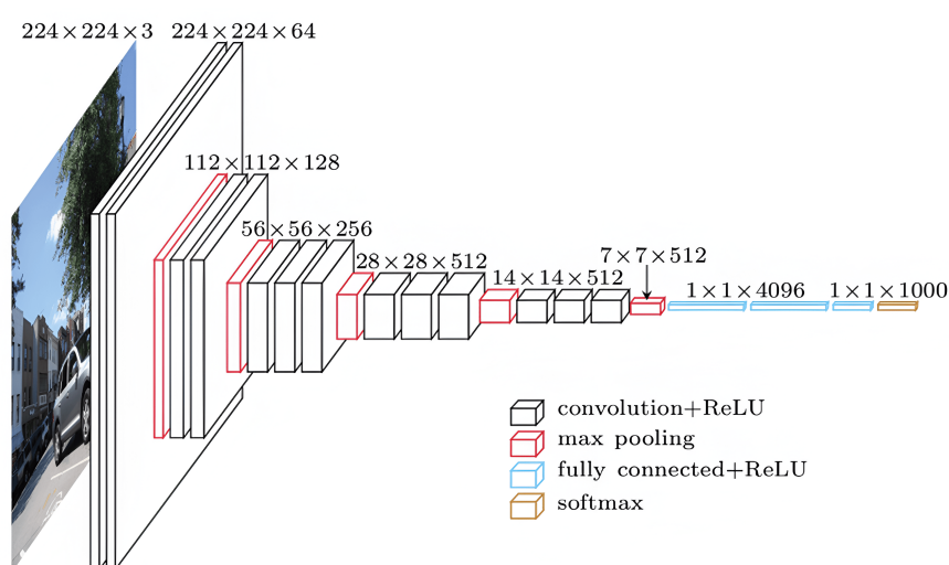
Figura 4.15: Arquitectura de la red VGG-16. Las dimensiones se muestran en formato: Columnas x Filas x Canales [76].
