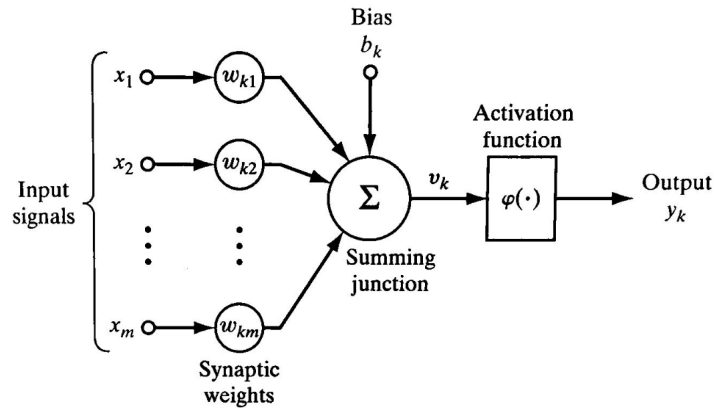
Figura 2.2: Diagrama detallado del modelo neuronal para una neurona k [40]. El diagrama muestra las señales de entrada que se multiplican por sus respectivos pesos. Estas señales ponderadas se suman junto con el sesgo, y se les aplica una función de activación para producir la salida de la neurona.
