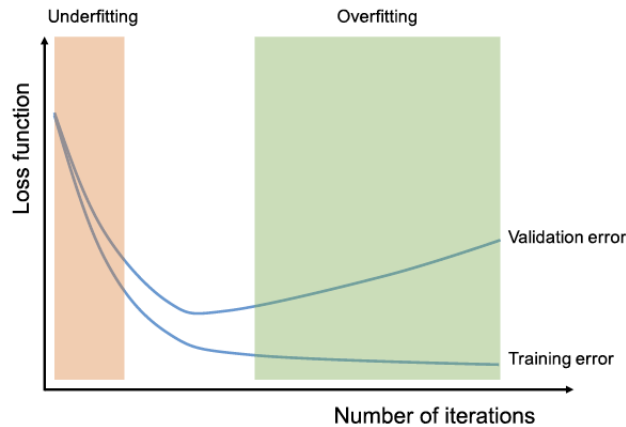
Figura 2.7: Zona de infraajuste y sobreajuste del modelo durante el entrenamiento [47]. El eje vertical representa la función de pérdida, mientras que el eje horizontal muestra el número de iteraciones durante el entrenamiento. Al inicio del proceso, tanto el error de entrenamiento como el de validación son altos, indicando que el modelo no ha aprendido lo suficiente de los datos, situación conocida como infraajuste. A medida que el entrenamiento avanza, ambos errores disminuyen hasta alcanzar un punto óptimo donde el modelo generaliza bien en datos no vistos. Sin embargo, si el entrenamiento continúa, el error de validación comienza a aumentar mientras que el error de entrenamiento sigue disminuyendo, fenómeno conocido como sobreajuste.
