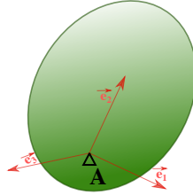
Figura 8: Sólido en movimiento de pivotamiento respecto de un punto A . El sistema de referencia en A está ligado al sólido.
