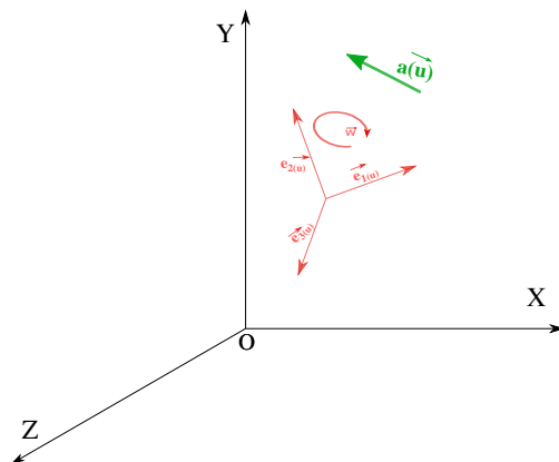
Figura 1: Ilustración de la Regla de Boure: Función vectorial \vec{a}(u) en función de un sistema de referencia móvil (en rojo) que depende del escalar u .
