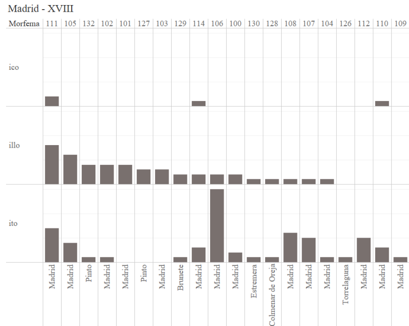
Figura 82: Dispersión de los diminutivos en el corpus de Madrid (s. XVIII)
