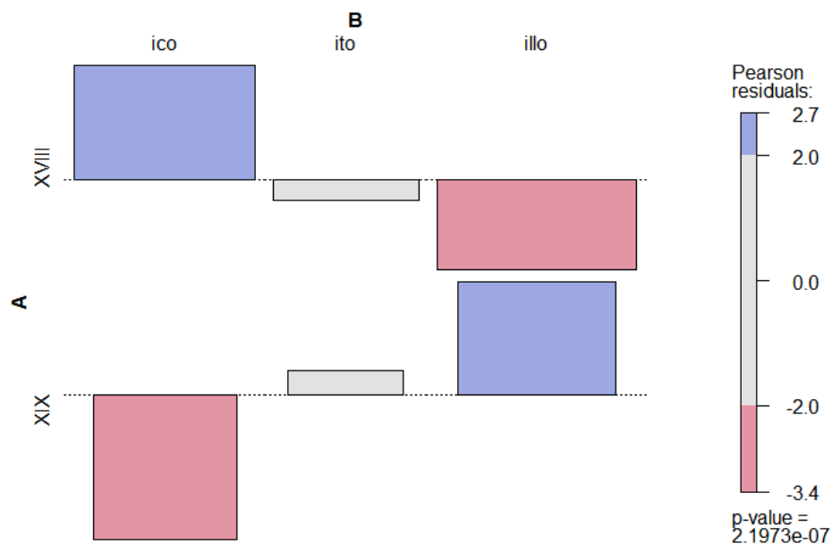
Figura 80: Asociación de las variables siglo/diminutivo en Almería basada en los residuos de Pearson
