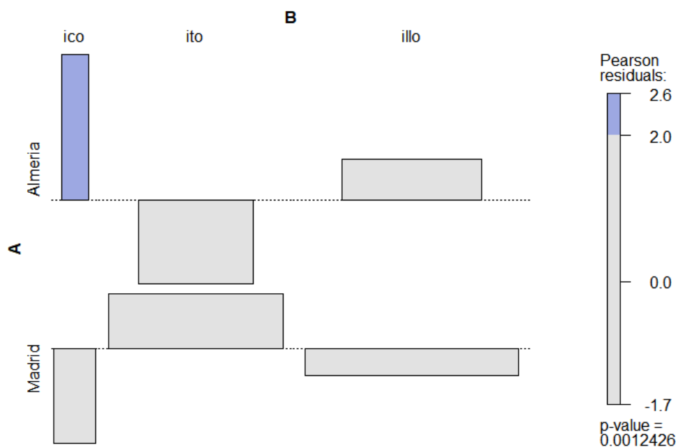
Figura 90: Gráfico de asociación (provincia/diminutivo en el s. XIX) basado en los residuos de Pearson
