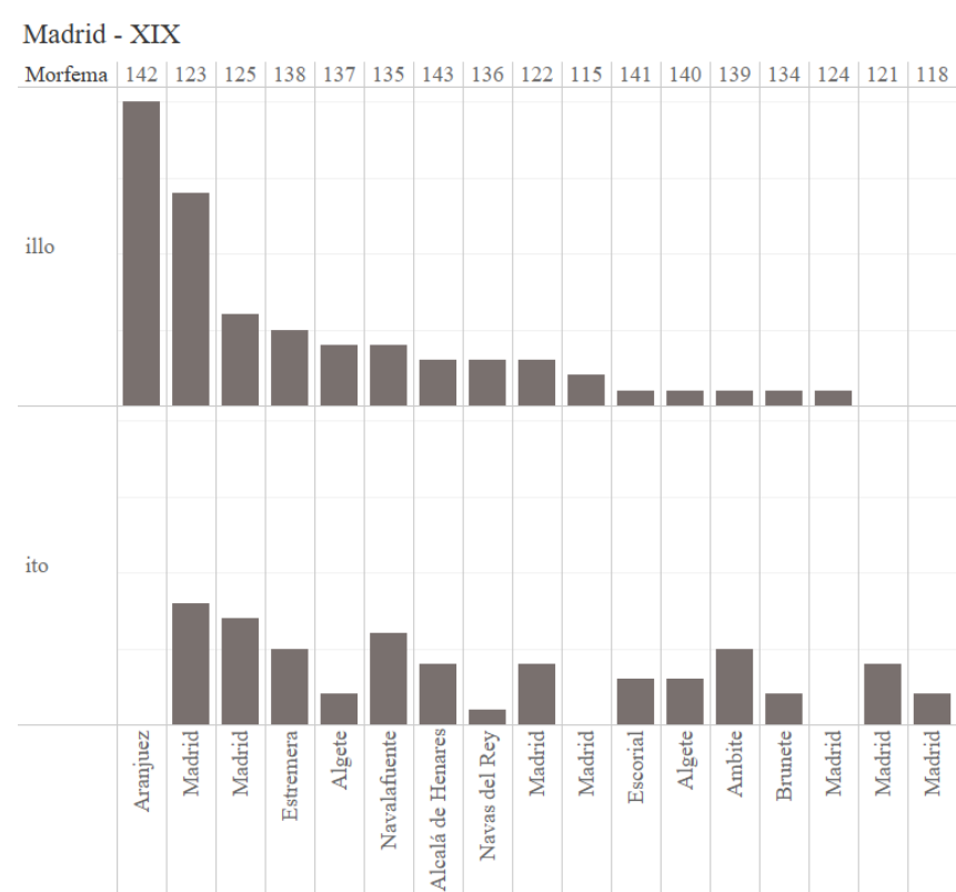
Figura 83: Dispersión de los diminutivos en el corpus de Madrid (s. XIX)
