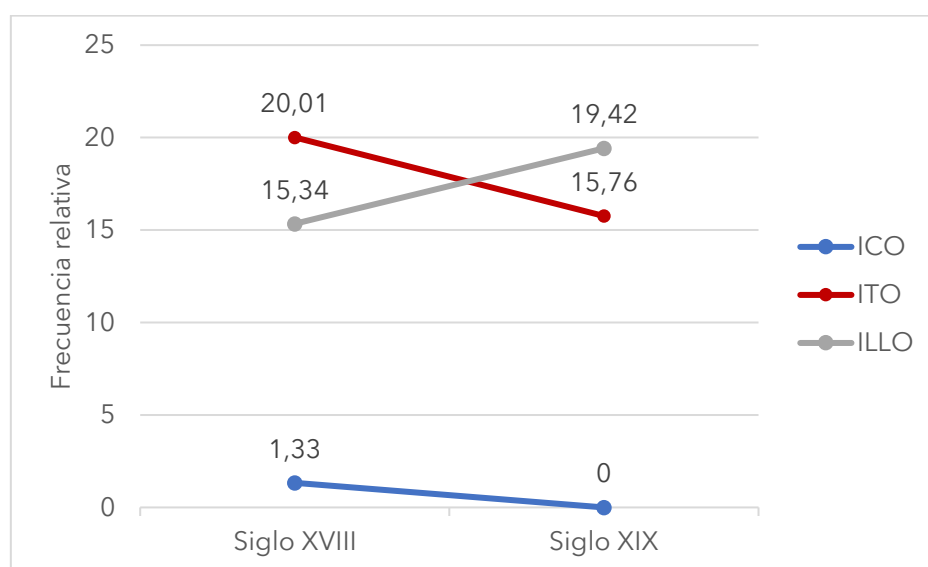
Figura 86: Distribución diacrónica de los diminutivos en Madrid en los siglos XVIII-XIX
