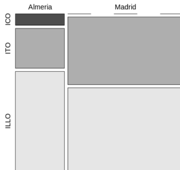
Figura 89: Proporción de uso de los diminutivos en Almería y Madrid en el s. XIX
