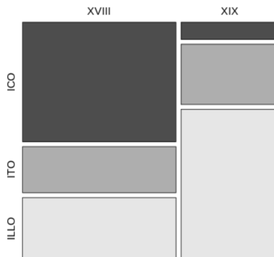
Figura 79: Distribución proporcional de los diminutivos en Almería en los ss. XVIII y XIX
