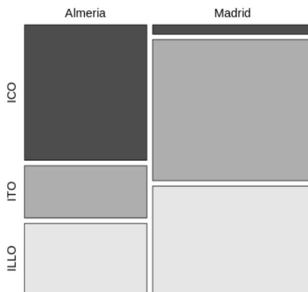
Figura 87: Proporción de los diminutivos en Almería y Madrid en el s. XVIII
