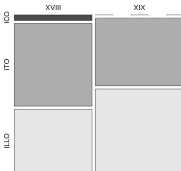
Figura 84: Distribución proporcional de los diminutivos en Madrid en los ss. XVIII y XIX
