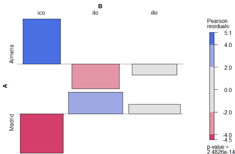
Figura 88: Gráfico de asociación (provincia/diminutivo en el s. XVIII) basado en los residuos de Pearson
