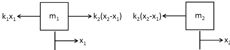
Figura 3.2 Diagrama de cuerpo libre. Sistema de 2 masas con 2 muelles en serie
