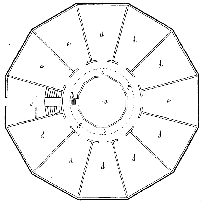
Panoptica de Jeremias Bentham.
