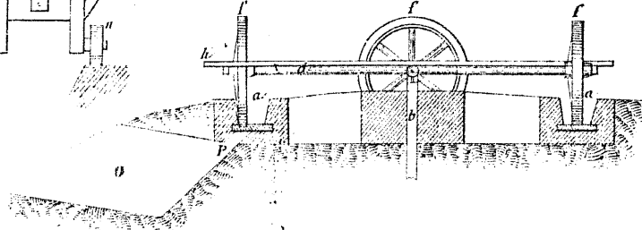
Corte.
