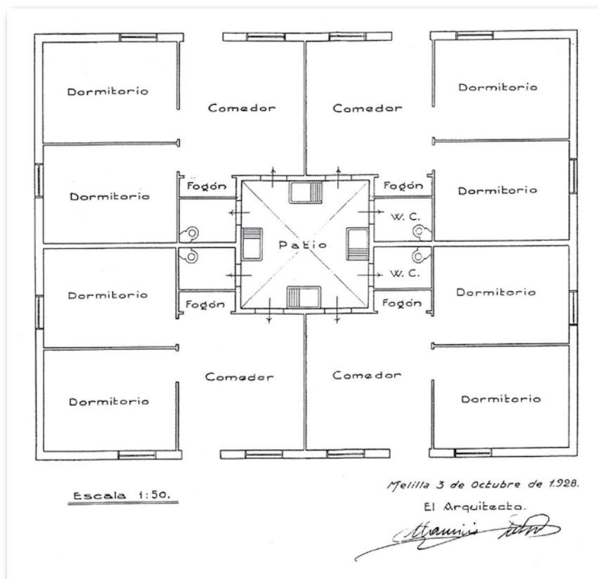
110. Viviendas del Barrio Primo de Rivera. Melilla. Planta. Arq. Mauricio Jalvo (3 de octubre de 1928). Archivo Central de Melilla. (SGA)
