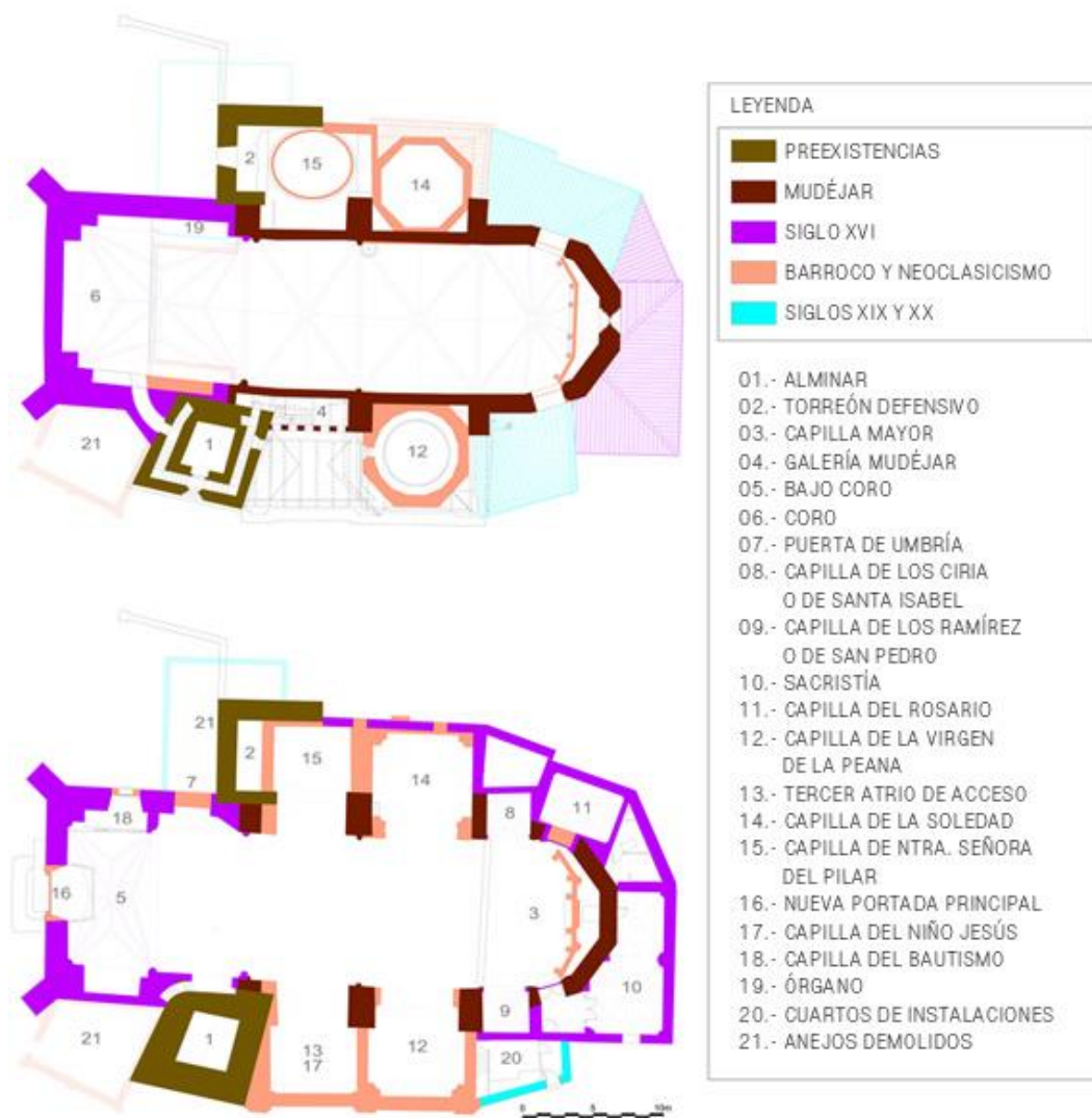
Ilustración 04. Plantas baja y a nivel del coro, con las distintas etapas constructivas, antes de las restauraciones. Fuente: Elaboración propia.
