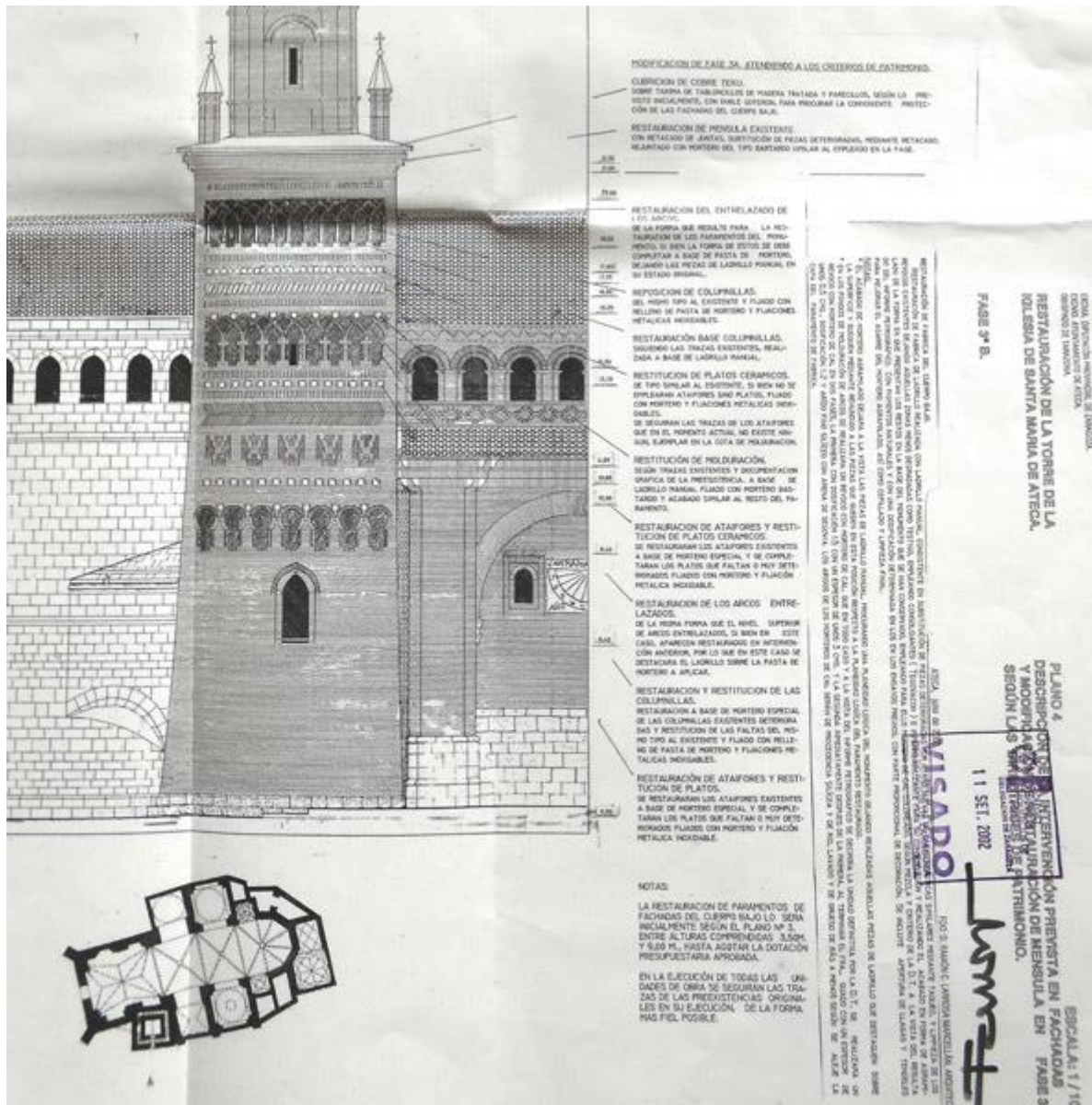
Link 16. “Restauración de la torre de la iglesia de Santa María de Ateca. Fase 3ª B, Plano 4. Descripción de la intervención prevista en fachadas y modificación de restauración de ménsula en fase 3 A”, Rafael Mérida Poch, julio de 2002 (visado el 11 de septiembre de 2002). Expediente 342/2002, Archivo de la Comisión Provincial de Patrimonio Cultural del Gobierno de Aragón.
