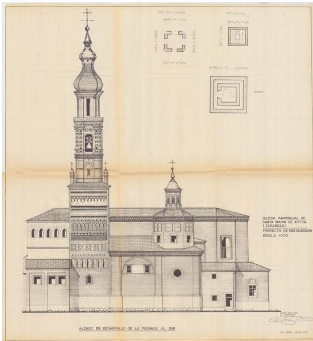
Alzado sur del edificio, reflejando el estado previo a la restauración. “Alzado en desarrollo de la fachada al sur.” Plano a escala 1/100 del Proyecto de restauración para la Iglesia Parroquial de Santa María de Ateca (Zaragoza). Rafael Mélida Poch, 1969. Archivo General de la Administración, (03)115.000, 26/00147.
