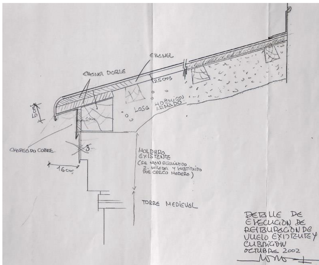
Link 18. “Detalle de ejecución de restauración de vuelo existente y cubrición. Octubre 2002”, Rafael Mélida Poch. Expediente 342/2002, Archivo de la Comisión Provincial de Patrimonio Cultural del Gobierno de Aragón.
