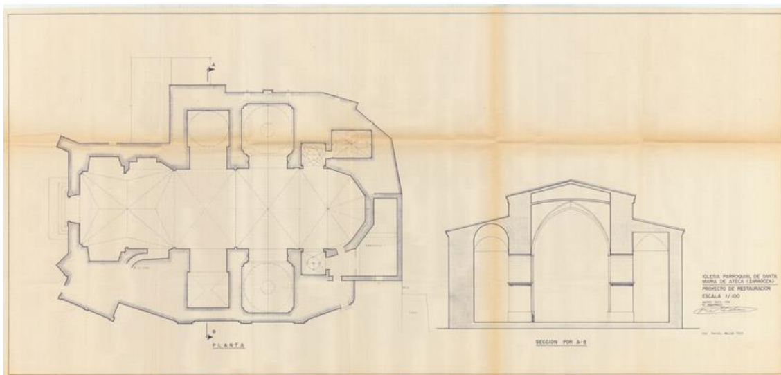
Link 03. Proyecto de restauración para la Iglesia Parroquial de Santa María de Ateca (Zaragoza), Plano de planta y sección a escala 1/100. Rafael Mélida Poch, 1969. Archivo General de la Administración, (03)115.000, 26/00147.
