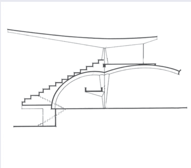
Gradas del Hipódromo de la Zarzuela. Imagen del voladizo exterior y sección (1935). Fuente: Archivo Torroja
