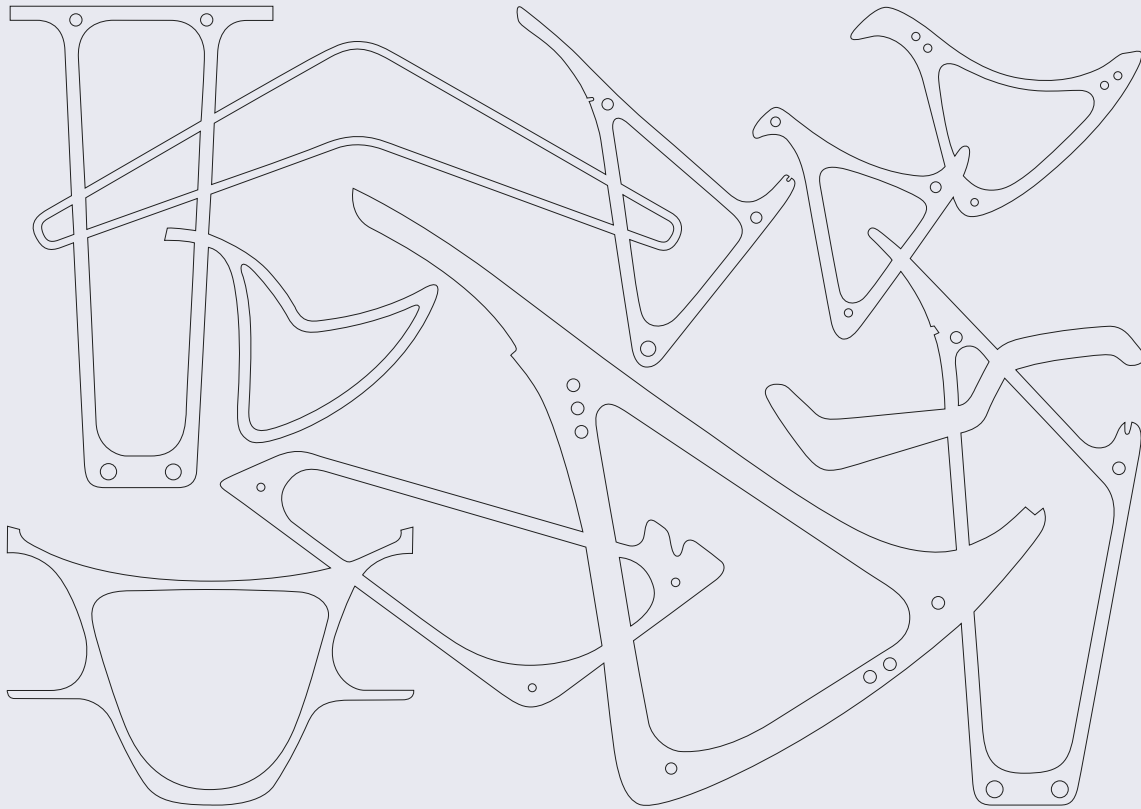
Perfiles de los "huesos" diseñados por Fisac entre 1960 y 1970. Fuente: exposición "Miguel Fisac. Huesos Varios". Ilustración de Mauro Doncel
