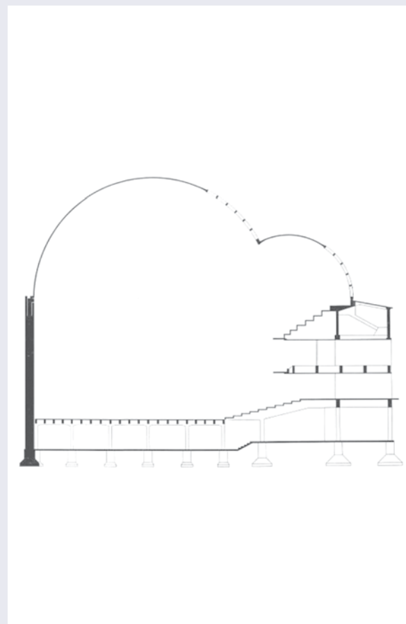
Gradas del Hipódromo de la Zarzuela. Imagen del voladizo exterior y sección (1935). Fuente: Archivo Torroja
