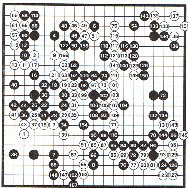
Ilustración 24: Partida de go que sirve a Jacques Roubaud para confeccionar uno de los cuatro itinerarios de lectura de Ε .
