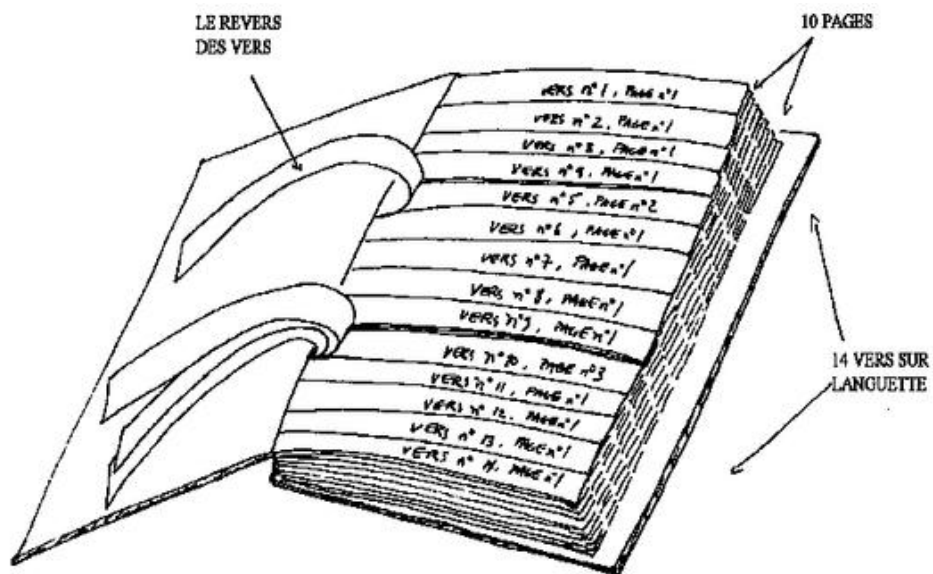
Ilustración 6: Modo de empleo de los Cent mille milliards de poèmes, según la edición original de Gallimard.
