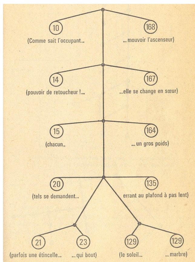
Ilustración 5: Gráfico arborescente que muestra la estructura de paréntesis encastrados de las Nouvelles impressions d'Afrique de Raymond Roussel.
