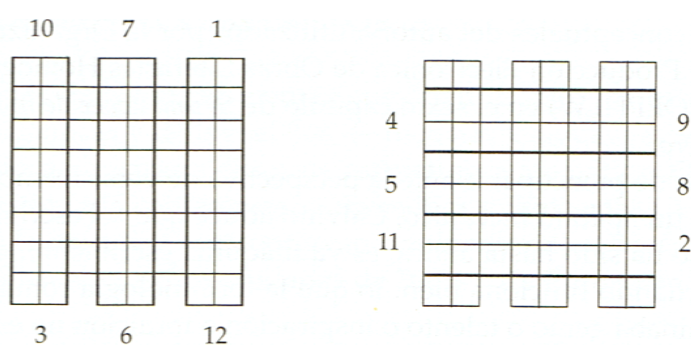
Ilustración 16: Esquema de las doce historias de El castillo .
