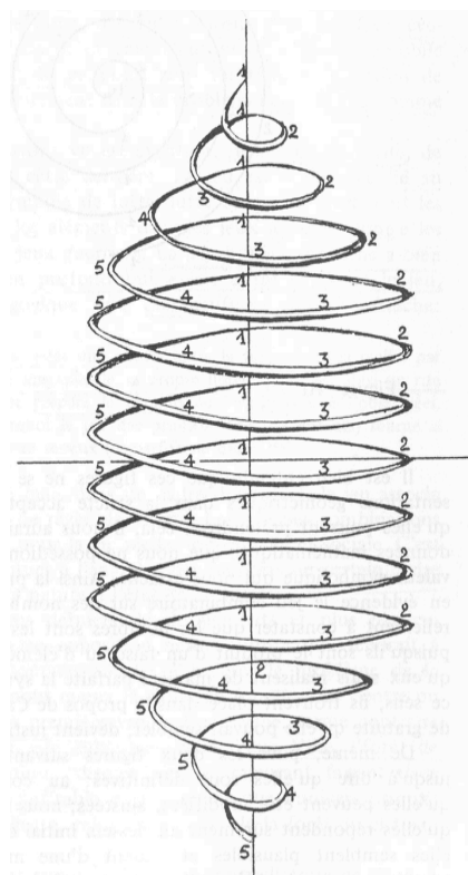
Ilustración 21: Estructura de Las ciudades invisibles según Aurore Frasson-Marin.
