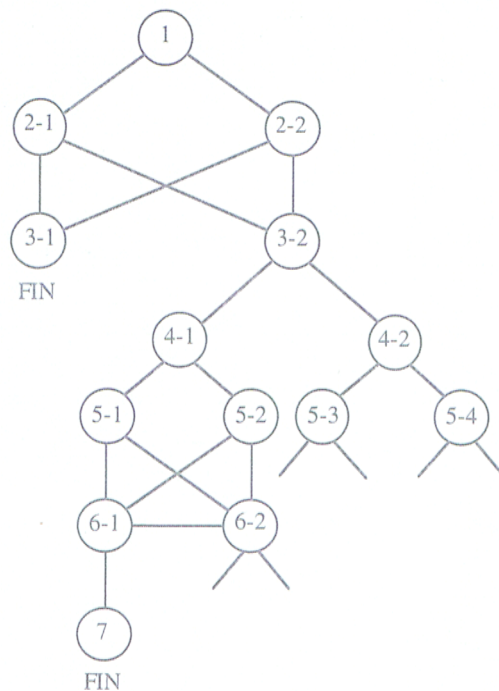
Ilustración 32: Estructura arborescente de Les premières heures de la colonie .
