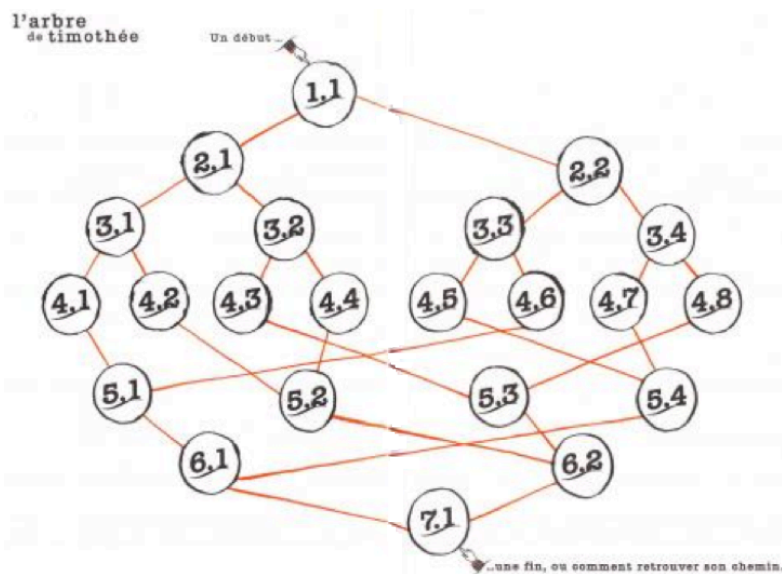
Ilustración 31: Grafo representativo de la estructura de Timothée dans l'arbre , de Paul Fournel.
