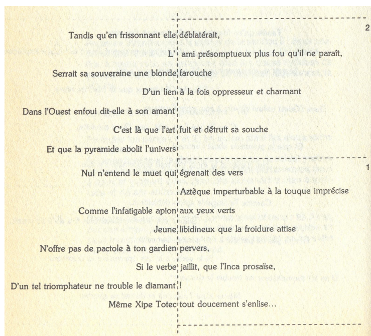
Ilustración 27b: Soneto «La princesse aztèque» en su versión de quinze versos.
