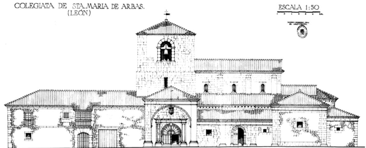
La colegiata de Santa María de Arbás, alzado general proyecto de restauración. Luis Menéndez-Pidal, 1964
