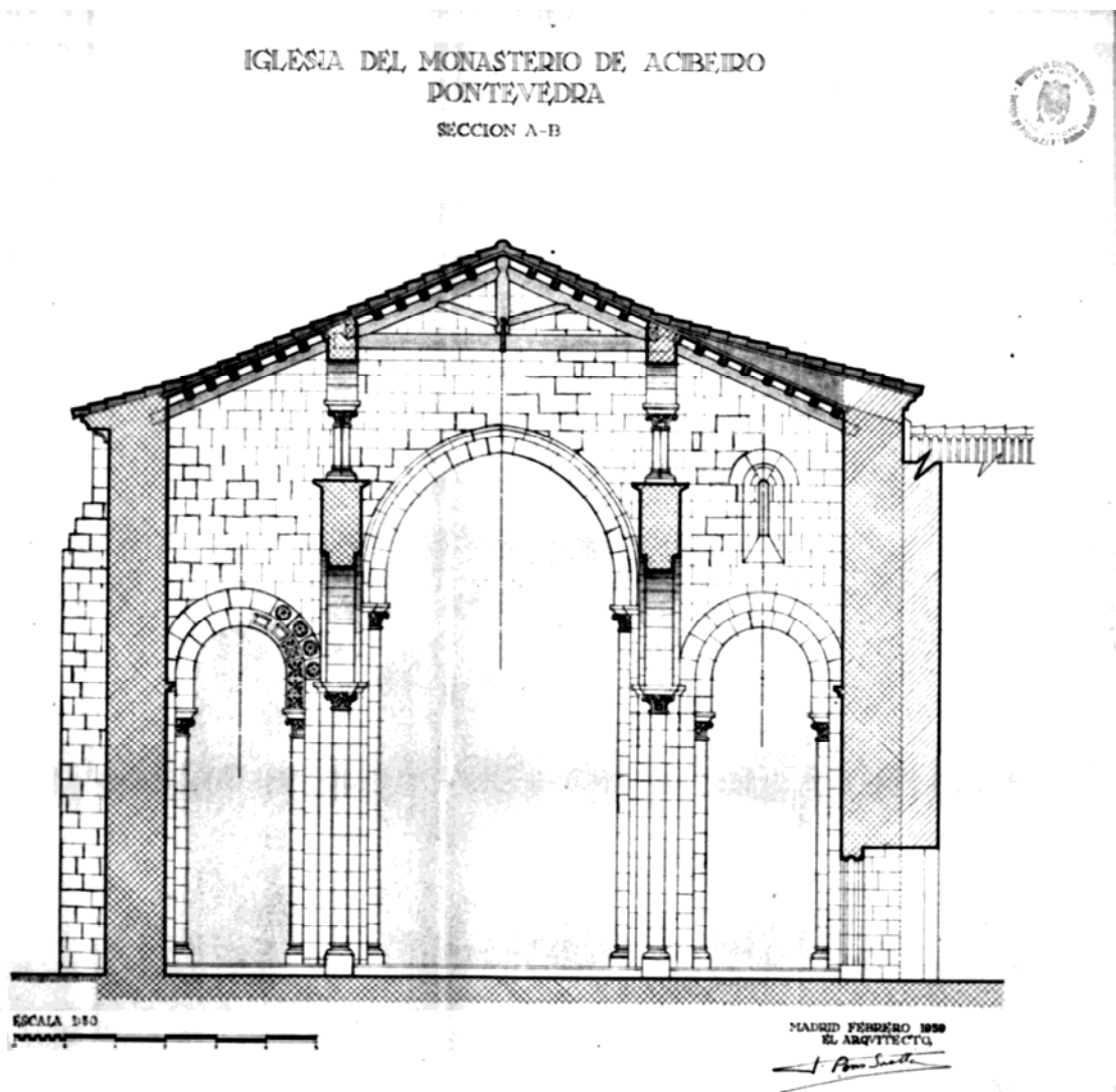
Iglesia del monasterio de Acibeiro, proyecto de restauración Luis Menéndez-Pidal y Francisco Pons Sorolla, 1947
