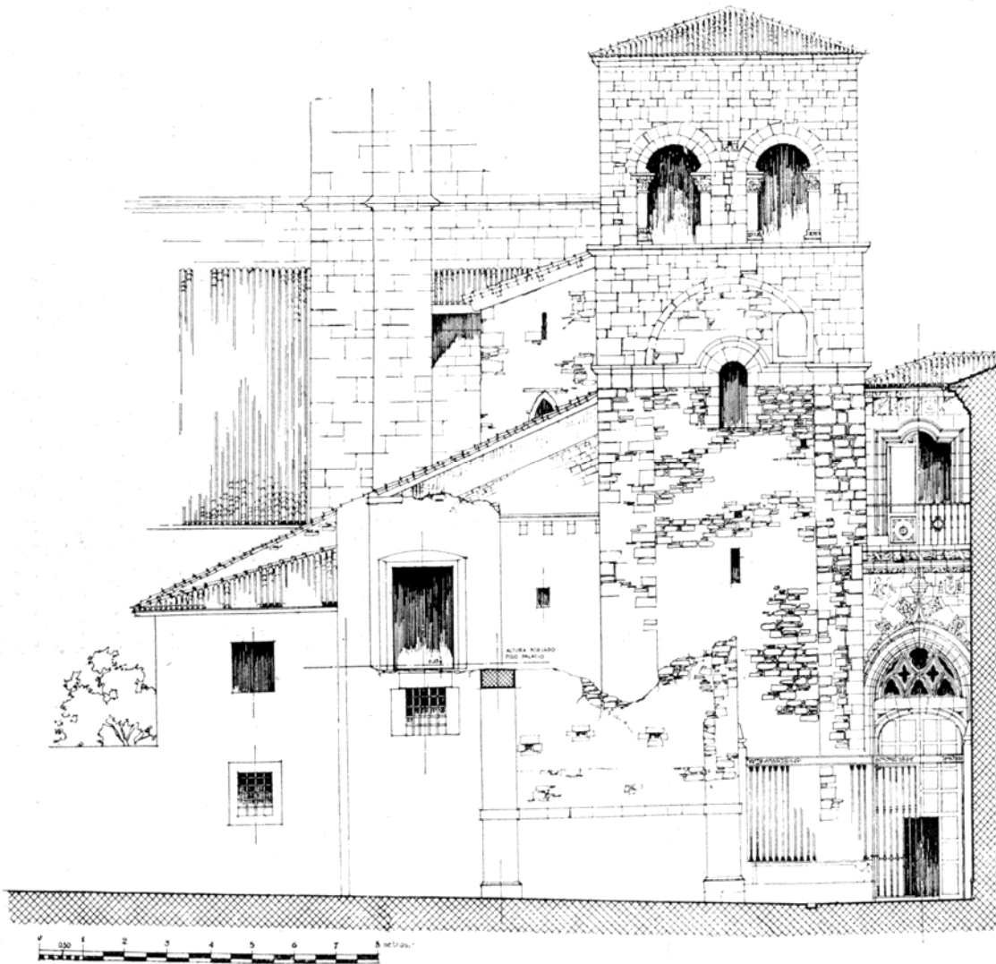
La torre Vieja de la catedral de Oviedo, estado previo tras la demolición del paso elevado. Luis Menéndez-Pida, 1951
