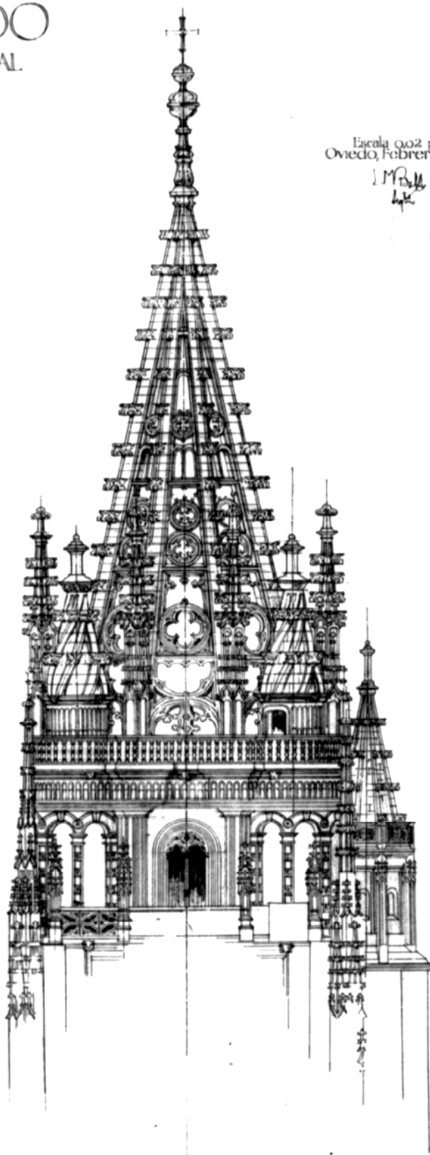
La torre Gótica de la catedral de Oviedo, proyecto de restauración Luis Menéndez-Pidal, 1944
