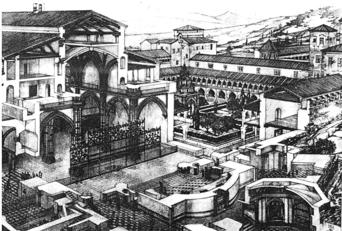
Monasterio de Guadalupe, sector de alzado principal (arriba) y axonometría seccionada, toma de datos del estado previo. Luis Menéndez-Pidal, 1933
