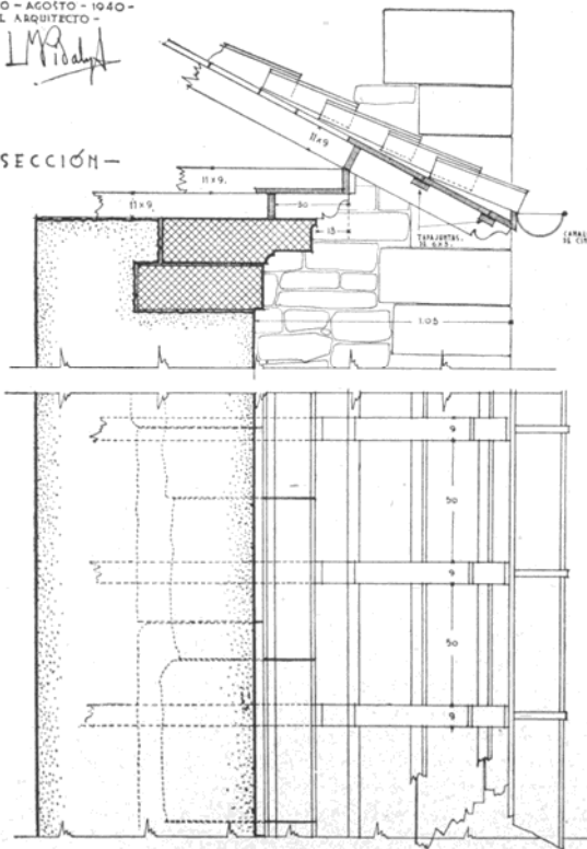
Detalle constructivo del alero del claustro del antiguo monasterio de San Vicente Luis Menéndez-Pidal, 1940
