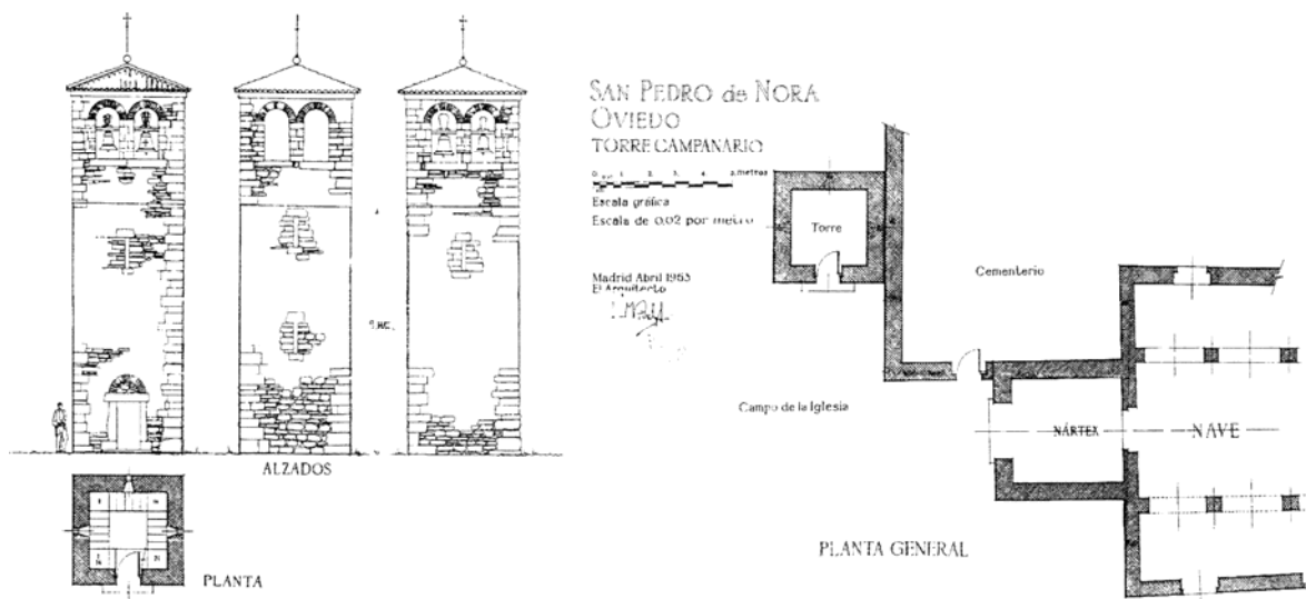
Proyecto para la nueva torre campanario de San Pedro de Nora Luis Menéndez-Pidal, 1957
