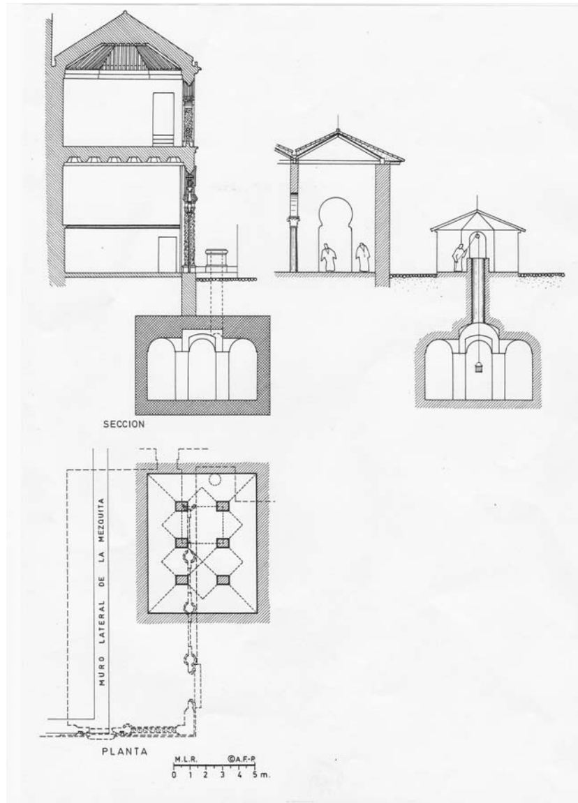
Fig. 3. Planta y sección del aljibe junto a la mezquita. Pabellón octogonal nazarí sobre el aljibe que cubría la fuente. (según M. López Bueno y P. Salmerón)
