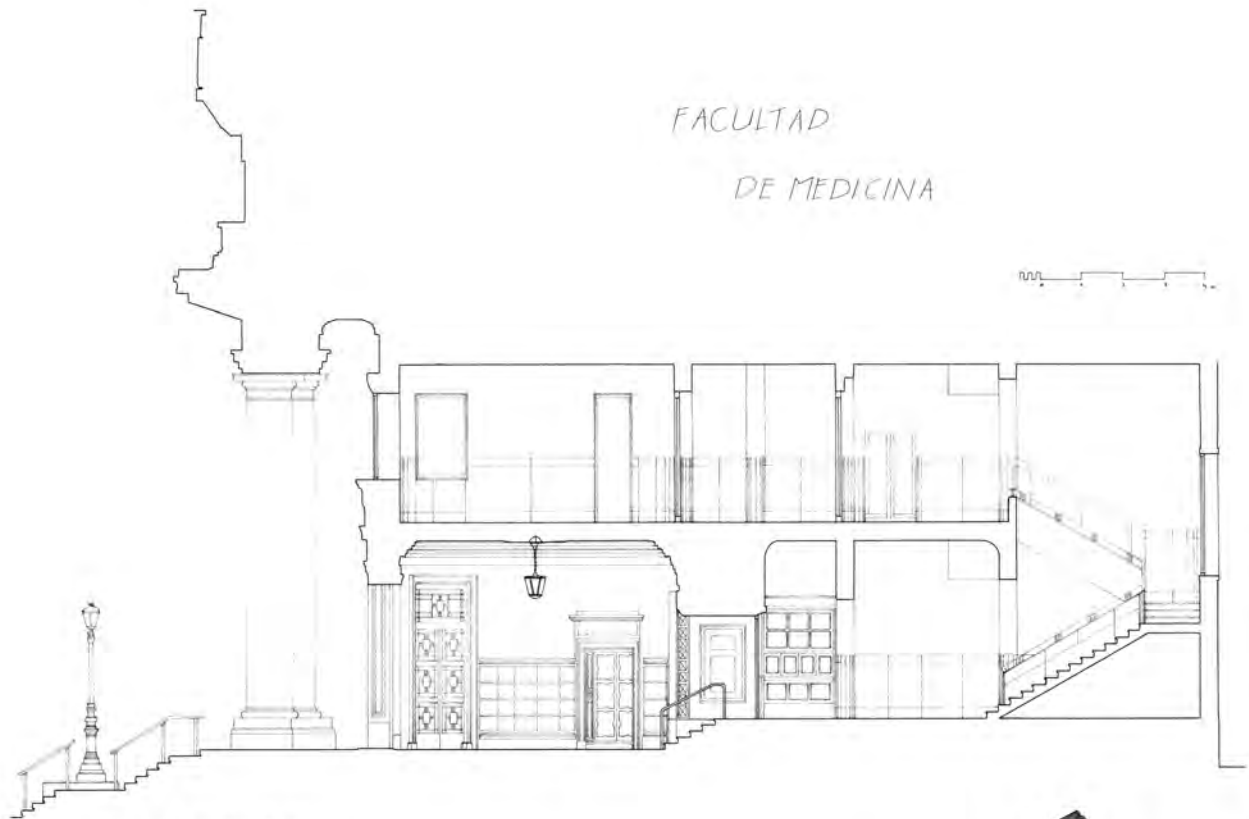
SECCION A-A
