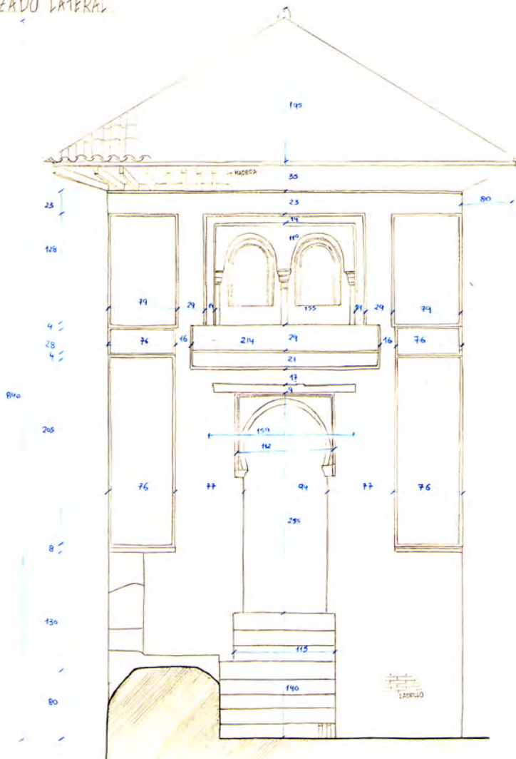
ALZADO LATERAL
