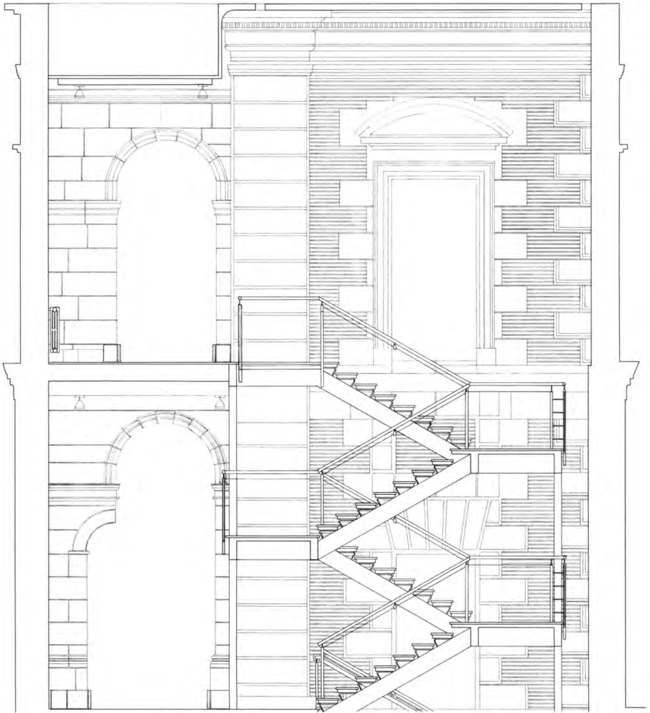
SECCION A-A
