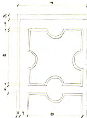
DETALLE B
