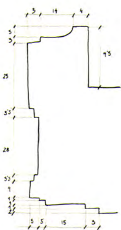
DETALLE A
