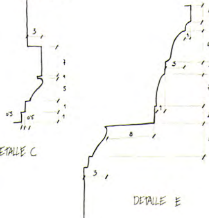
DETALLE D
