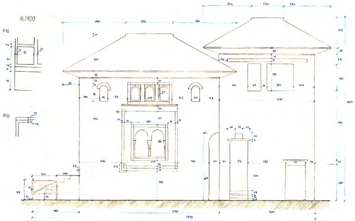
ALZADO LATERAL
