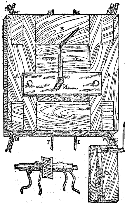
Nymphodori Glossocomum clausum.
