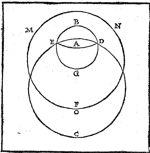
In hac figura sit .a. centrum terræ, quod est etiā centrum vniuersi, & sit sphaera terræ .b. d. g. e. super centrum .a. & sit sphaera aquæ .m. n. g. f. c.
