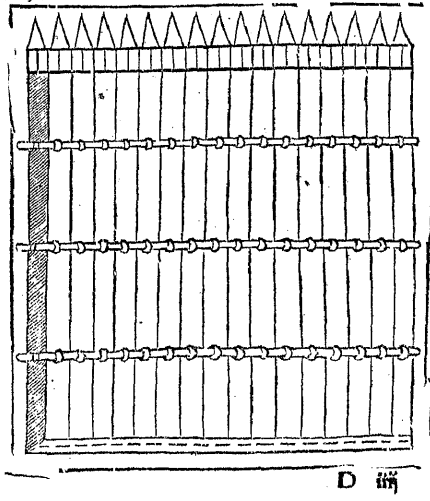
Sequitur figura vnus lateris taber- naculi, quantum ad tabulas es- bales quibus insiguntur.
