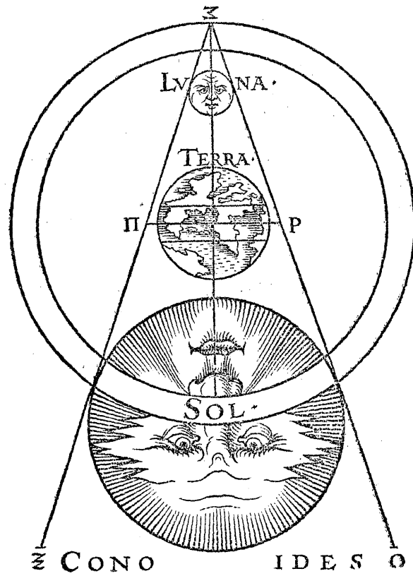
DE LVNA SOLE ET TERRA
