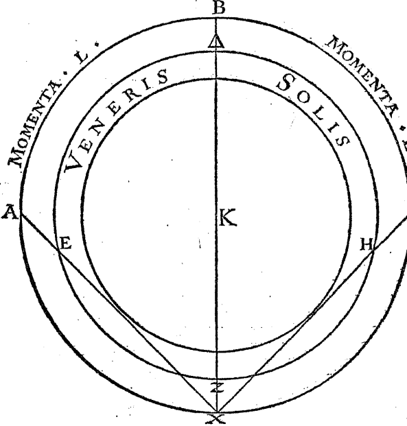
DE SOLE ET VENERE
