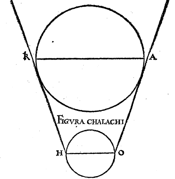
DE ECLYPSI OMIVM PLANETARVM.
