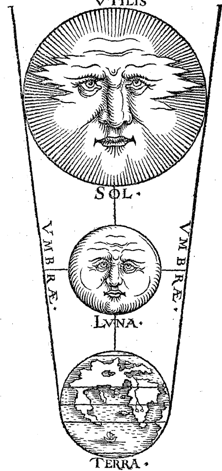
DE ECLYPSI SOLIS FIGVRA VUTILIS
