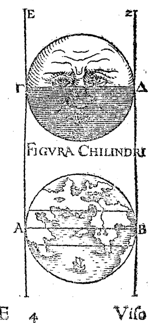
DE ECLYPSI LVNÆ
