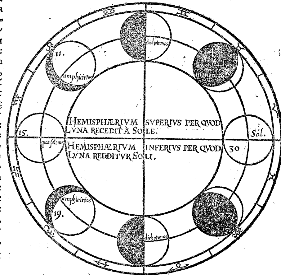
DE ECLYPSI LVNÆ
