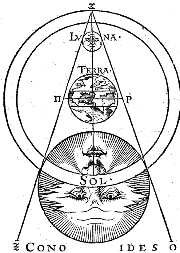
DE LVNA SOLE ET TERRA
