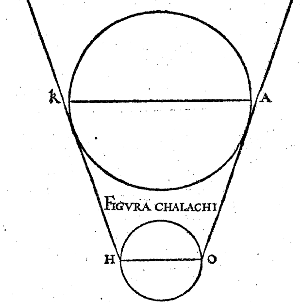
DE ECLYPSI OMIVM PLANETARVM
