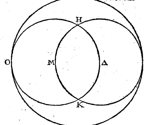
DE VNA ESSENTIA INNECTVNCVR SIBIDVO CIRCVLI
