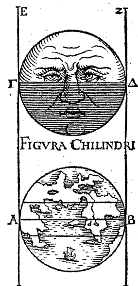
DE ECLYPSI OMIVM PLANETARVM
